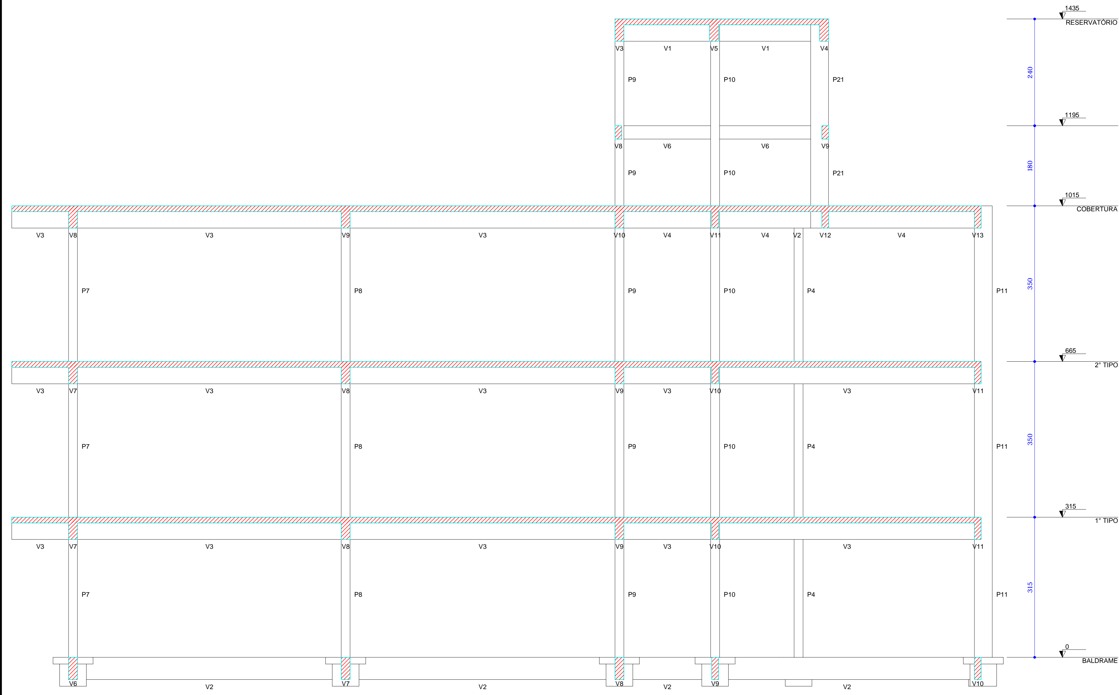
CORTE AA 1:50
