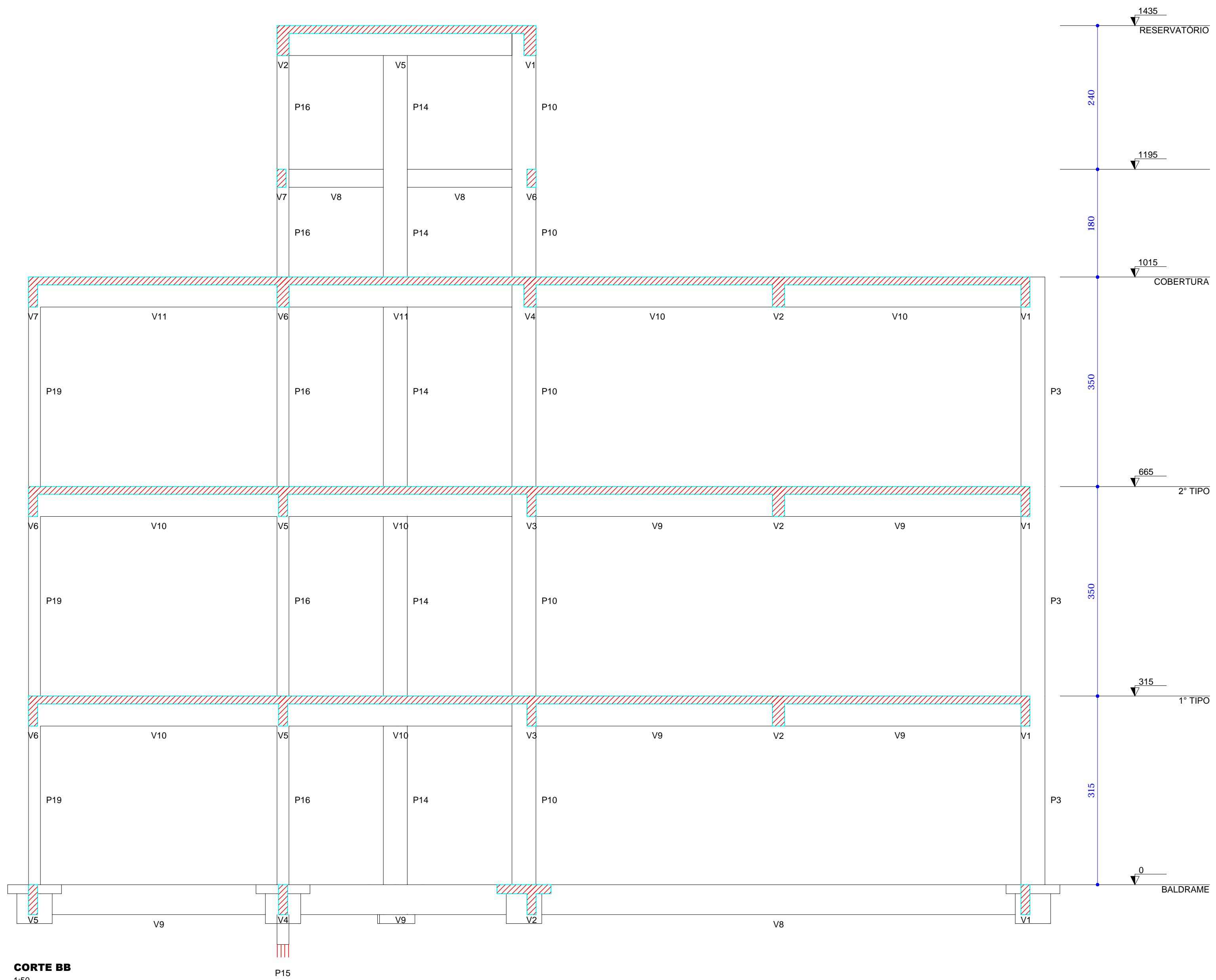
CORTE BB 1:50
