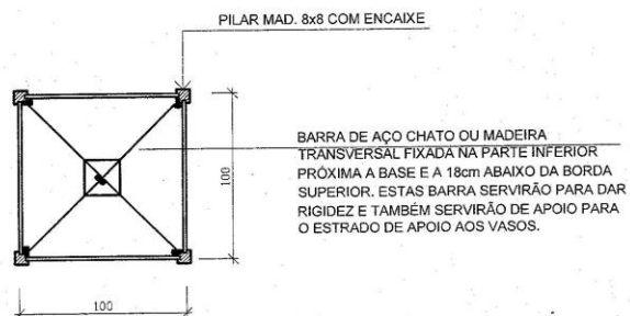
PLANTA BAIXA
