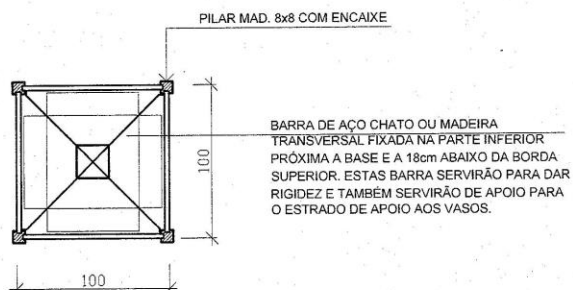
VISTA
