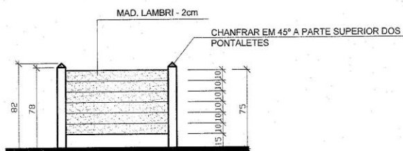
VISTA
