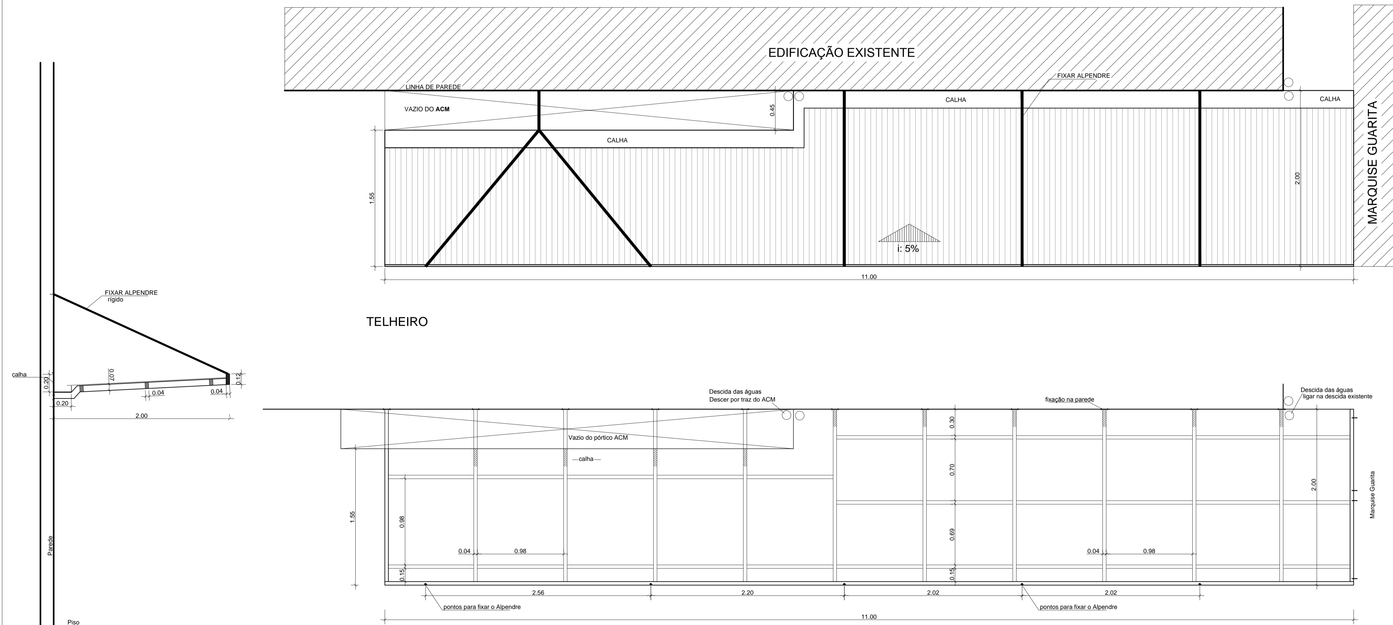
ESTRUTURA APOIO DE TELHAS
