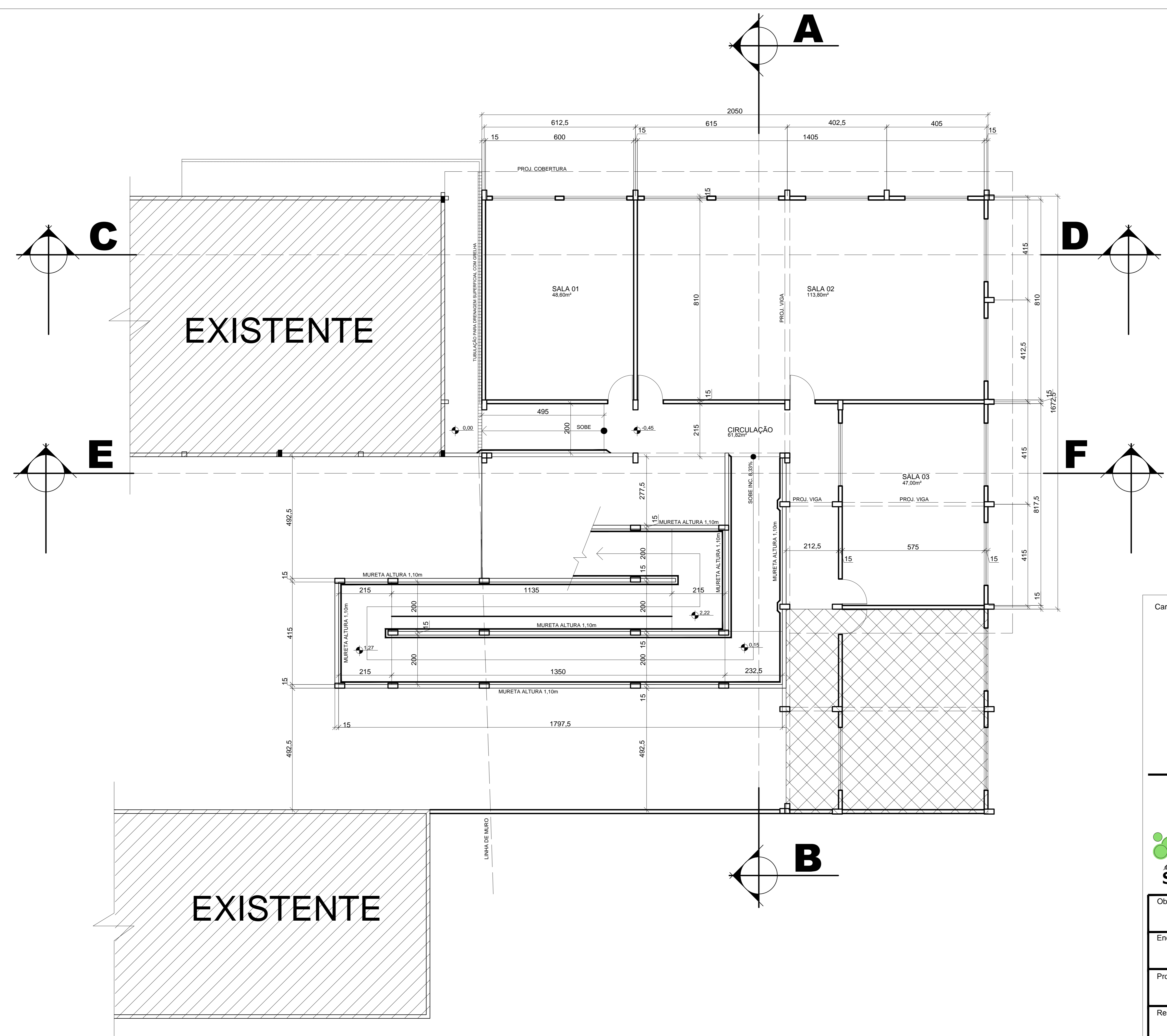
PLANTA BAIXA - SUBSOLO ESC.....1/75
