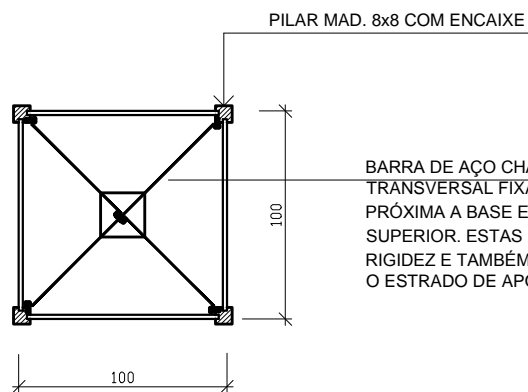
PLANTA BAIXA
