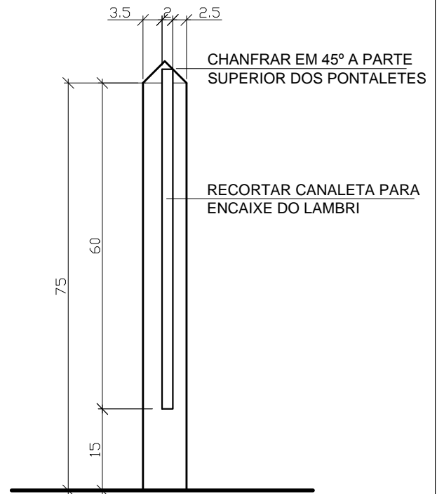
DETALHE CANALETA PILAR
