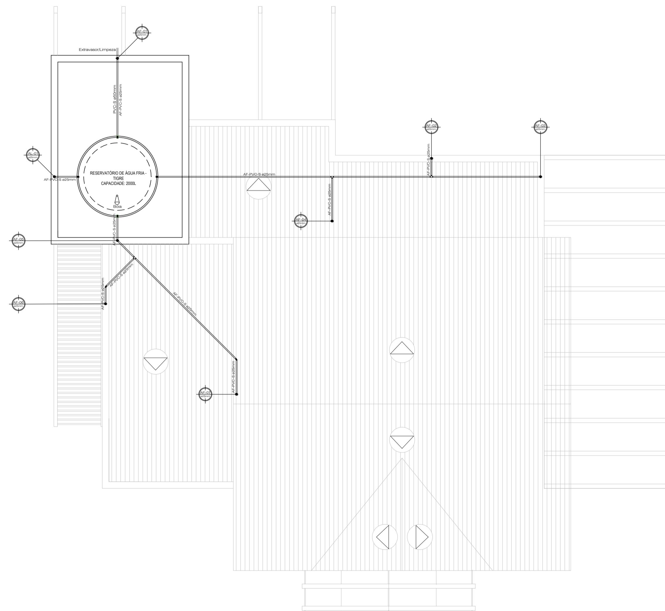
PLANTA DE COBERTURA HIDROSSANITÁRIO ESCALA: 1/50
