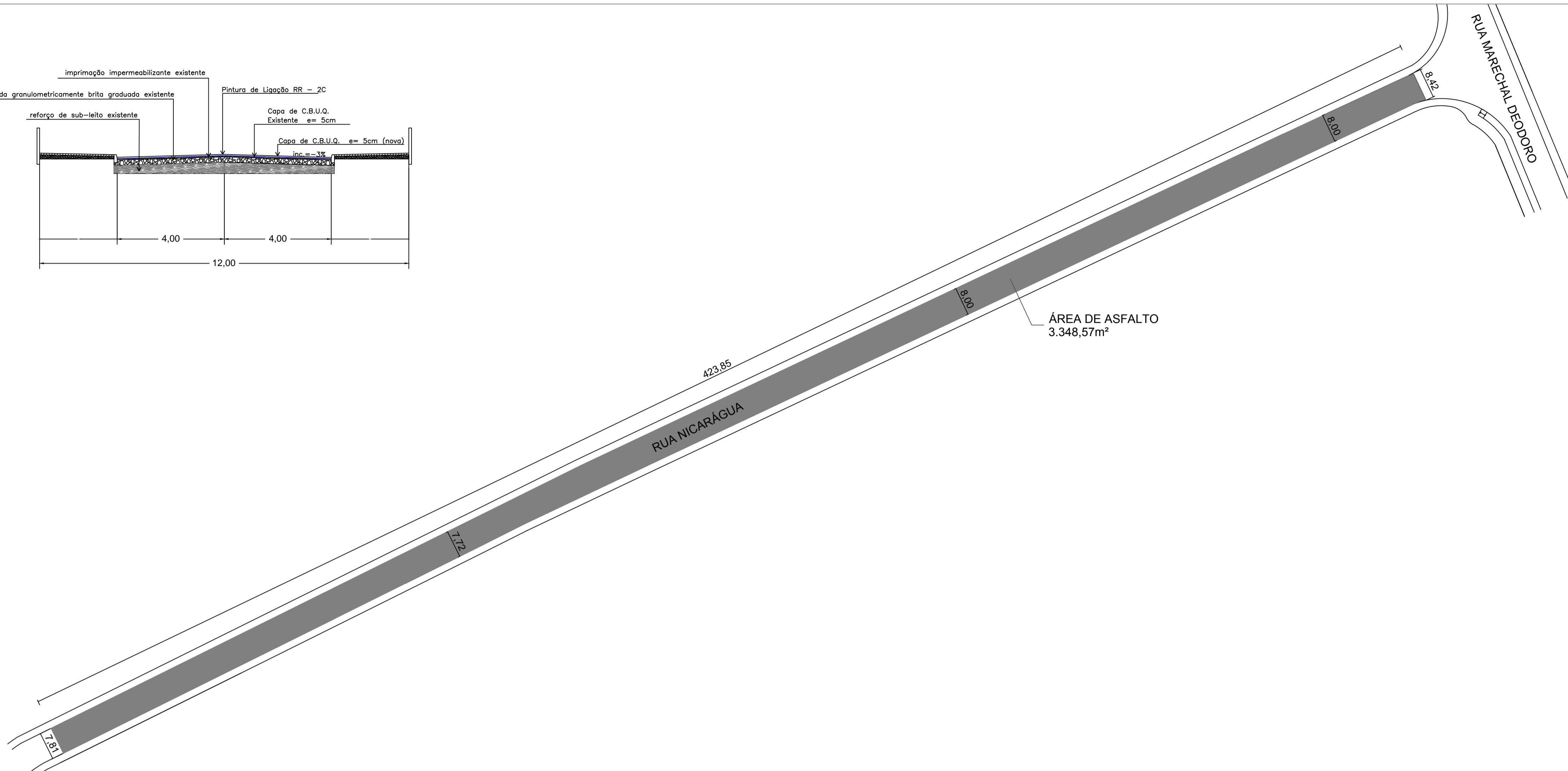
PLANTA DE PAVIMENTAÇÃO ESCALA 1:750
