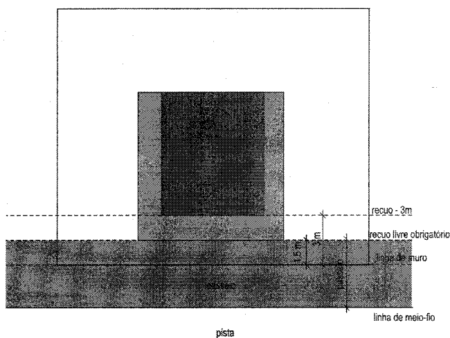
PLANTA BAIXA
