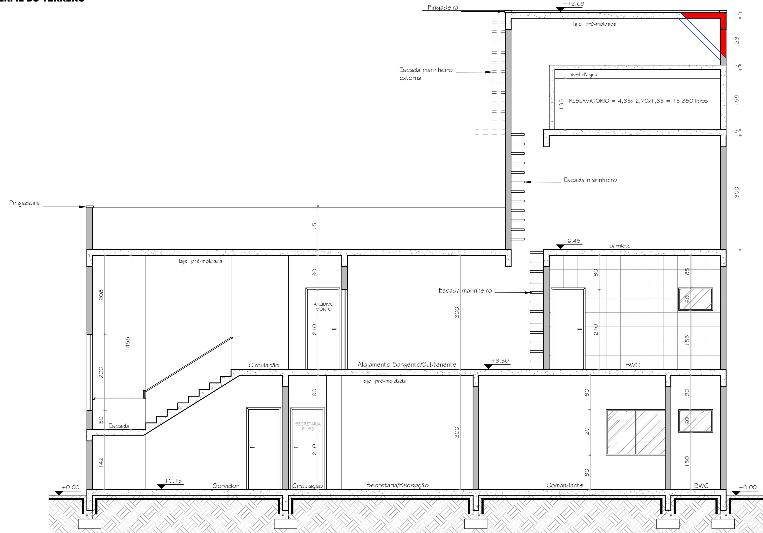
CORTE BB 1:50
