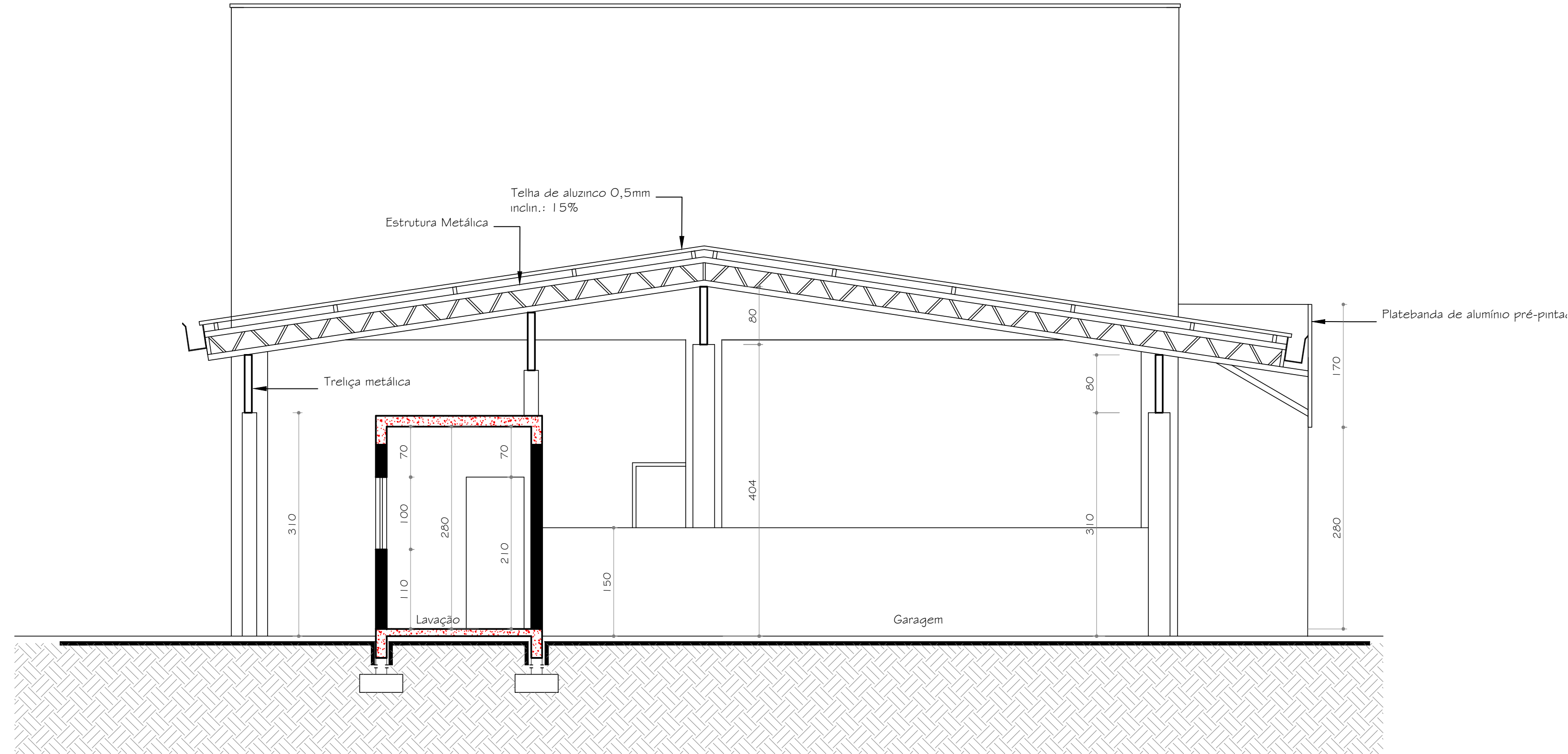
CORTE DD 1:50
