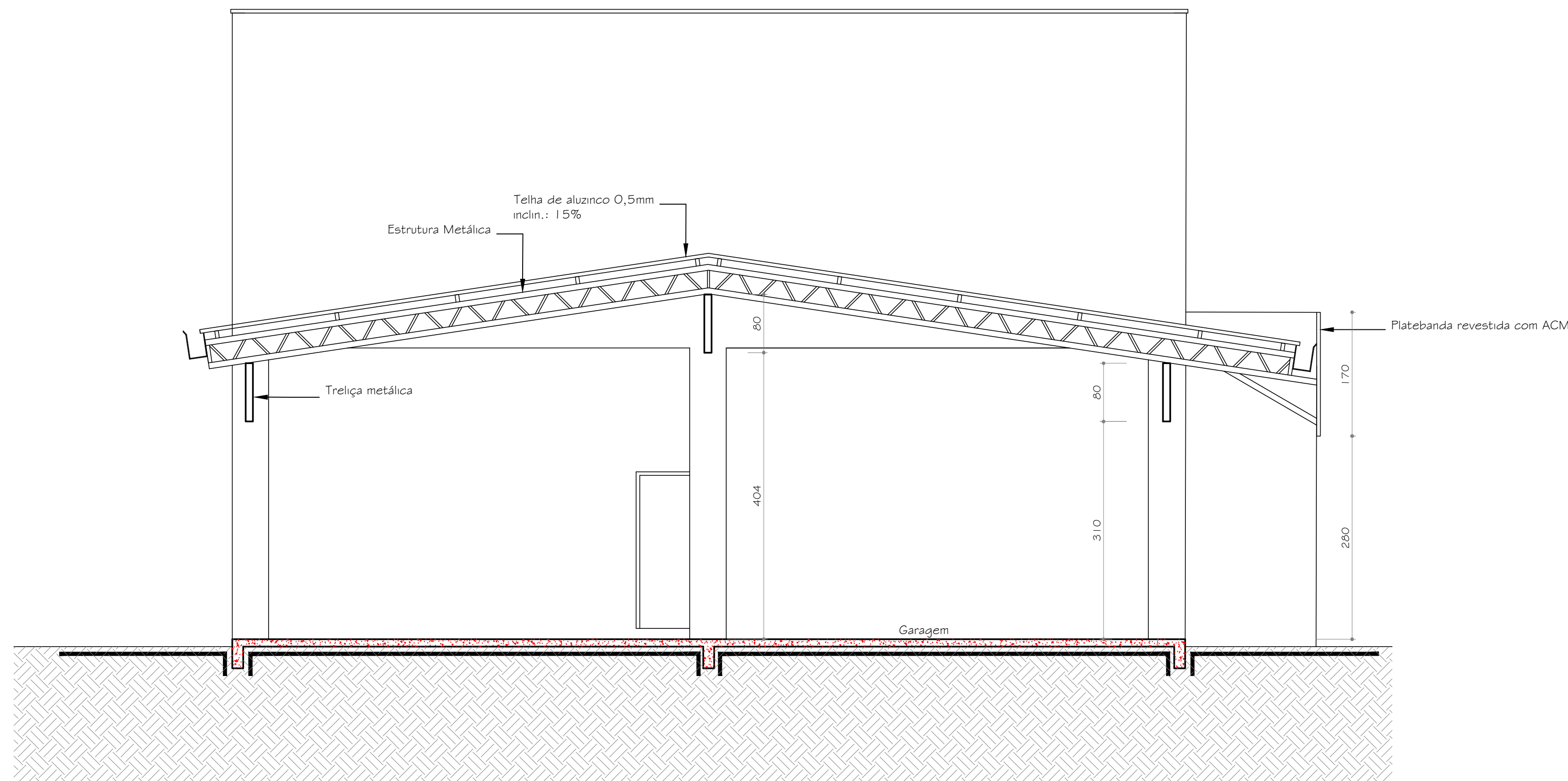
CORTE CC 1:50
