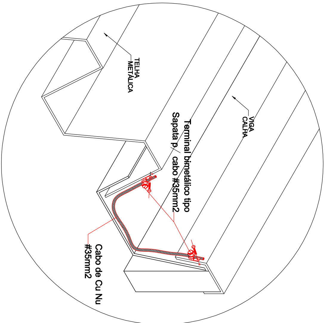
06 SEM ESCALA DETALHE INTERLIGAÇÃO DOS TELHADOS COM CABOS DE CU NU #35mm²
