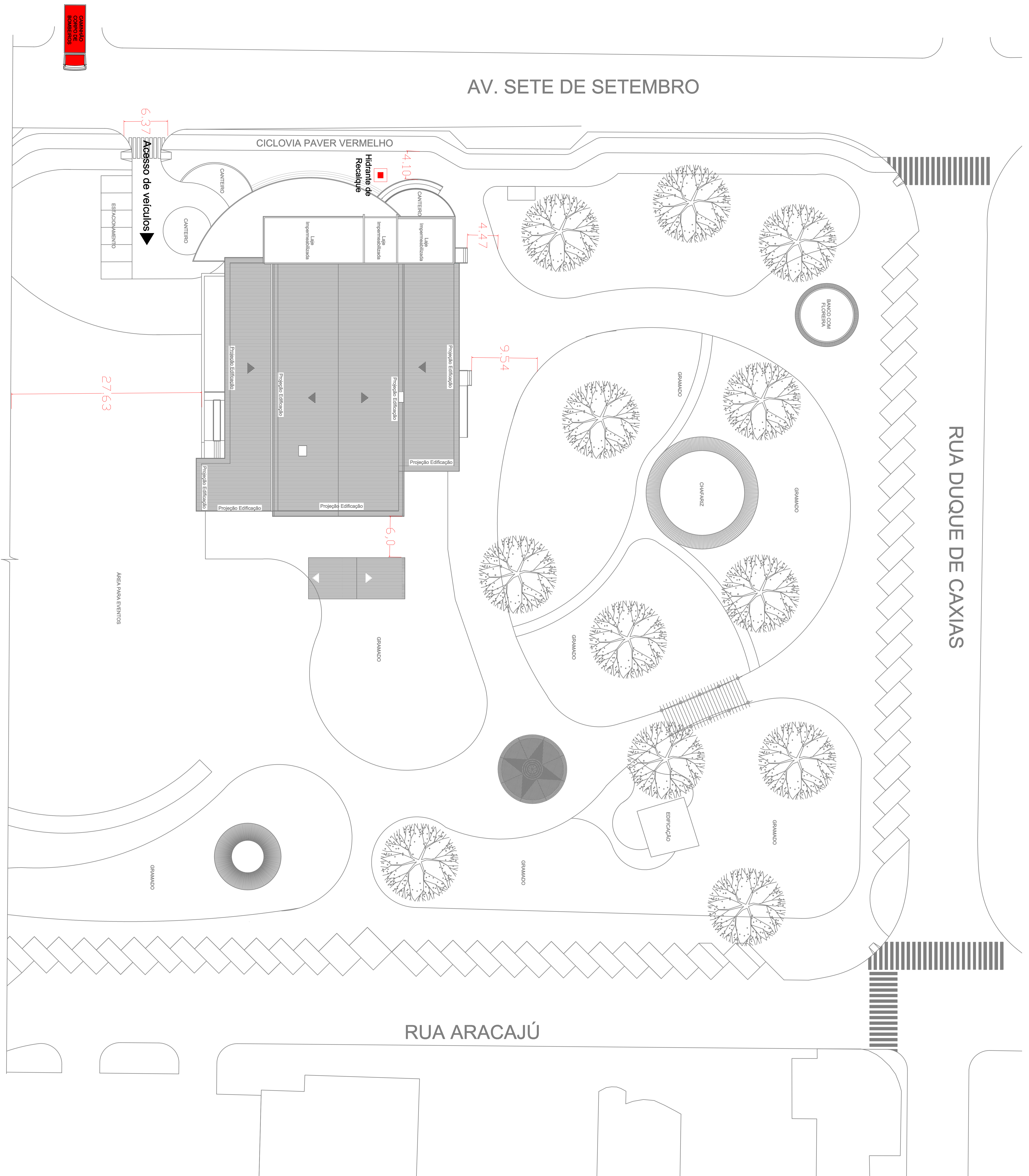
01 PLANTA DE SITUAÇÃO ESCALA 1:200
