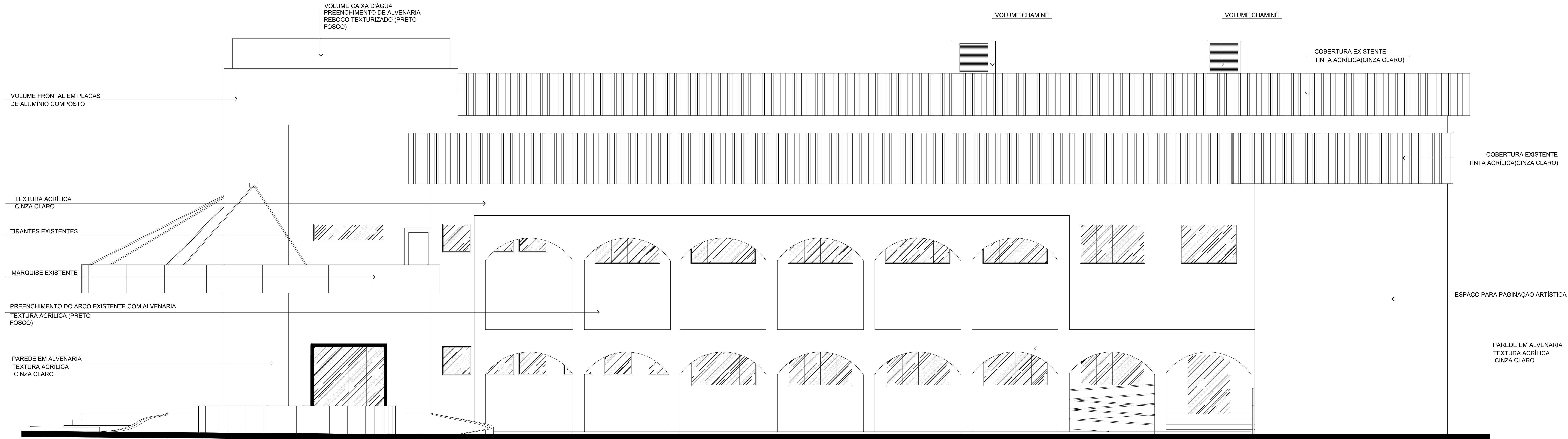
15 Fachada lateral sul Escala 1:50
