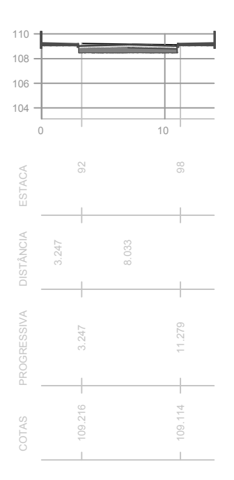
PERFIL TRANSVERSAL 04
