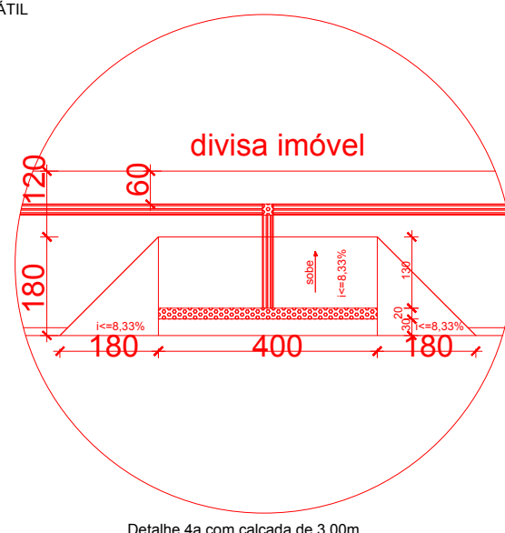
Detalhe 4a com calçada de 3,00m
