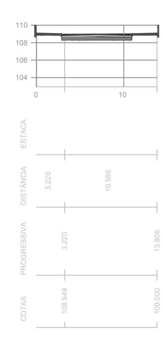
PERFIL TRANSVERSAL 03
