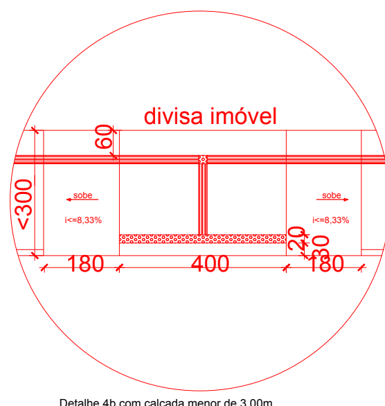
Detalhe 4b com calçada menor de 3,00m
