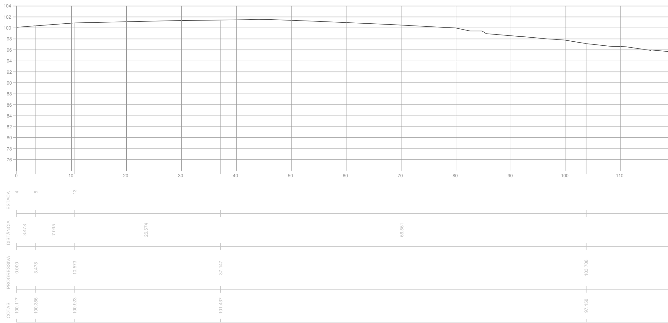
PERFIL LONGITUDINAL EIXO "RUA SÃO PAULO"
