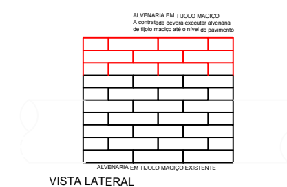
ALTEAMENTO DAS CAIXAS COLETORAS
