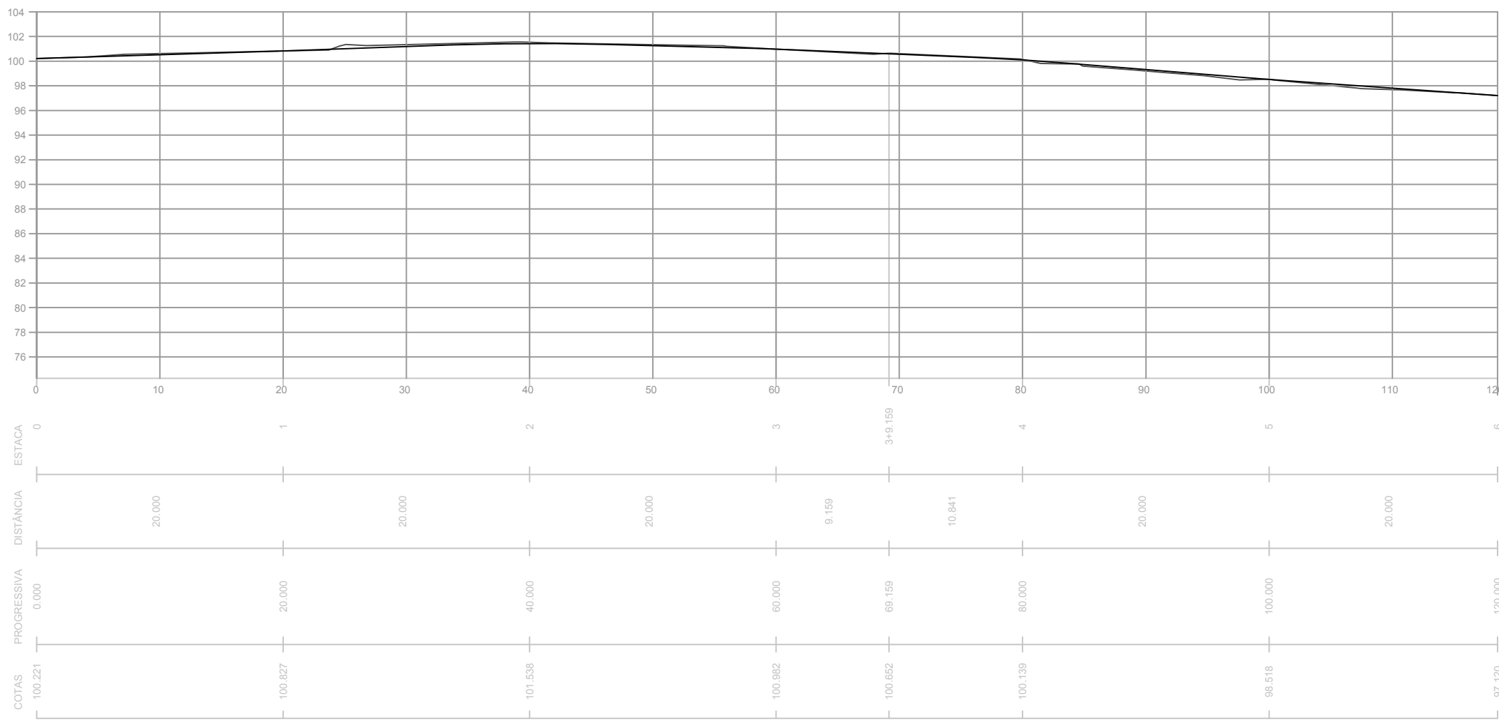
PERFIL LONGITUDINAL LADO ÍMPAR "RUA SÃO PAULO"
