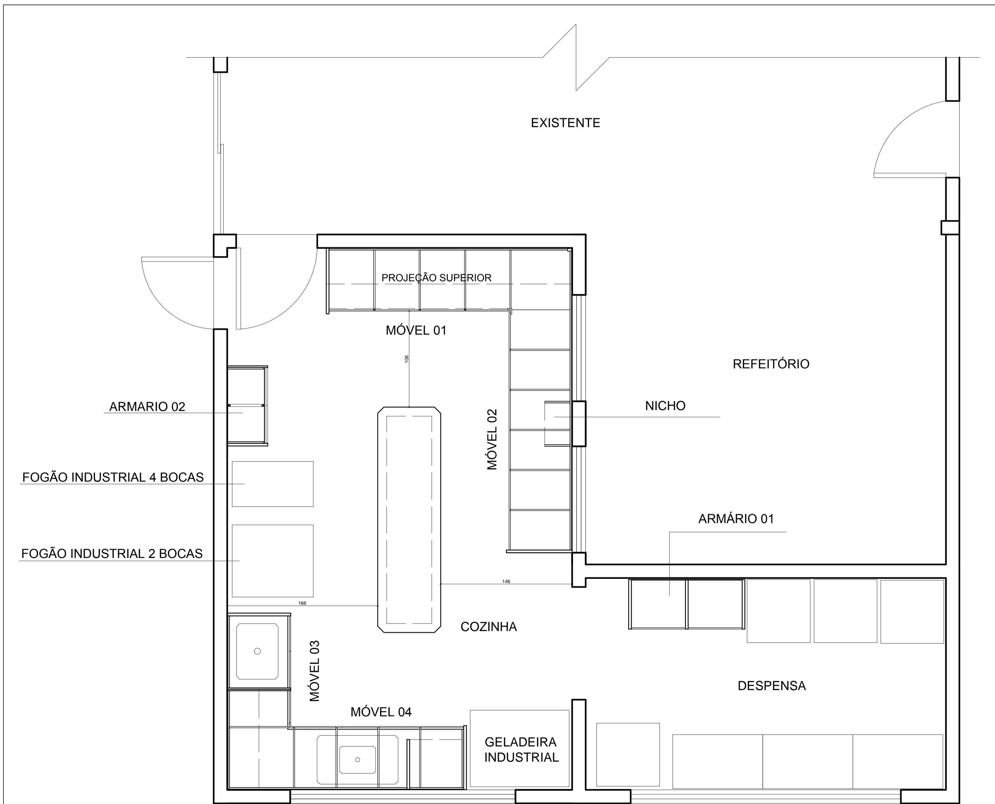
PLANTA BAIXA COZINHA ESCALA 1:25
