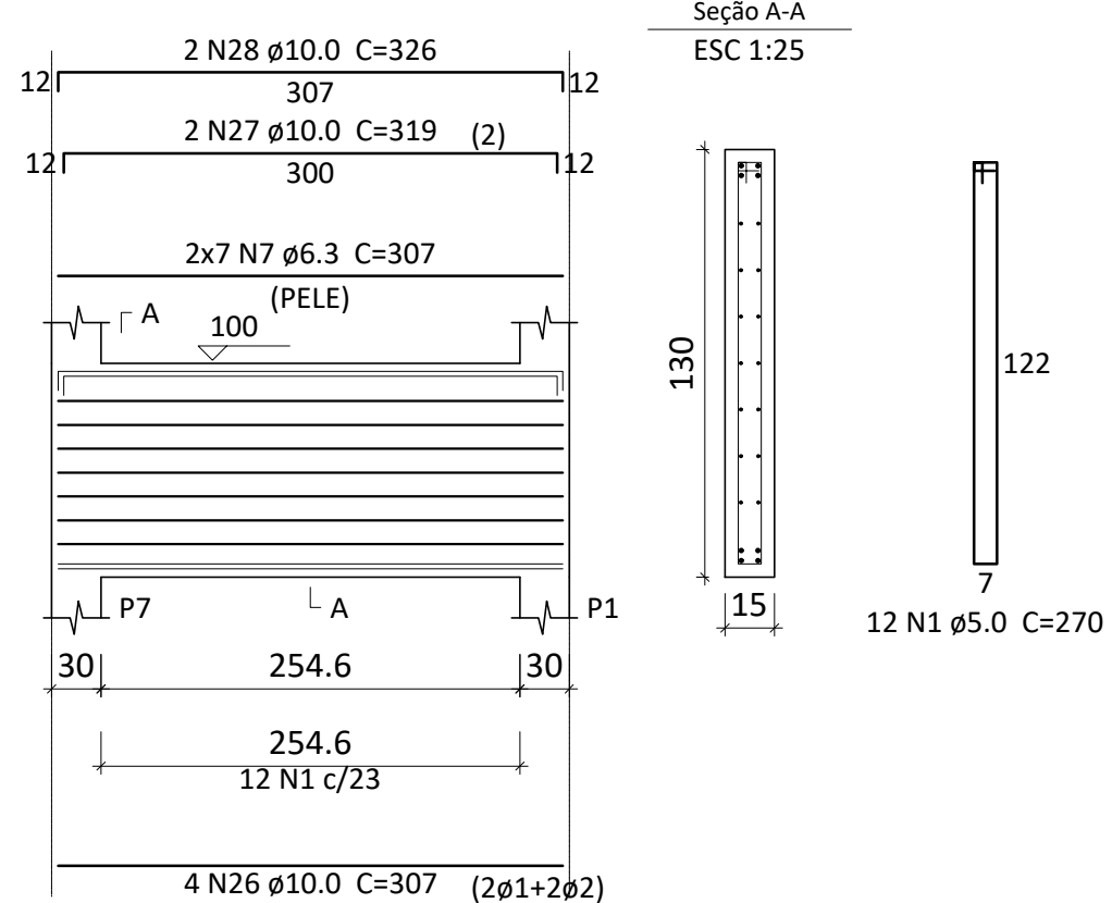
V11 ESC 1:50
