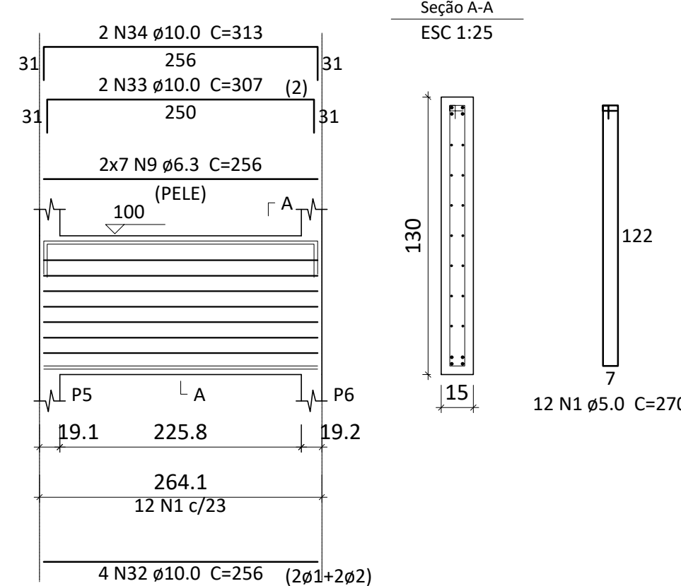
V13 ESC 1:50
