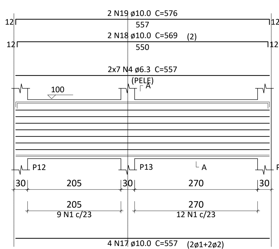
V5 ESC 1:50
