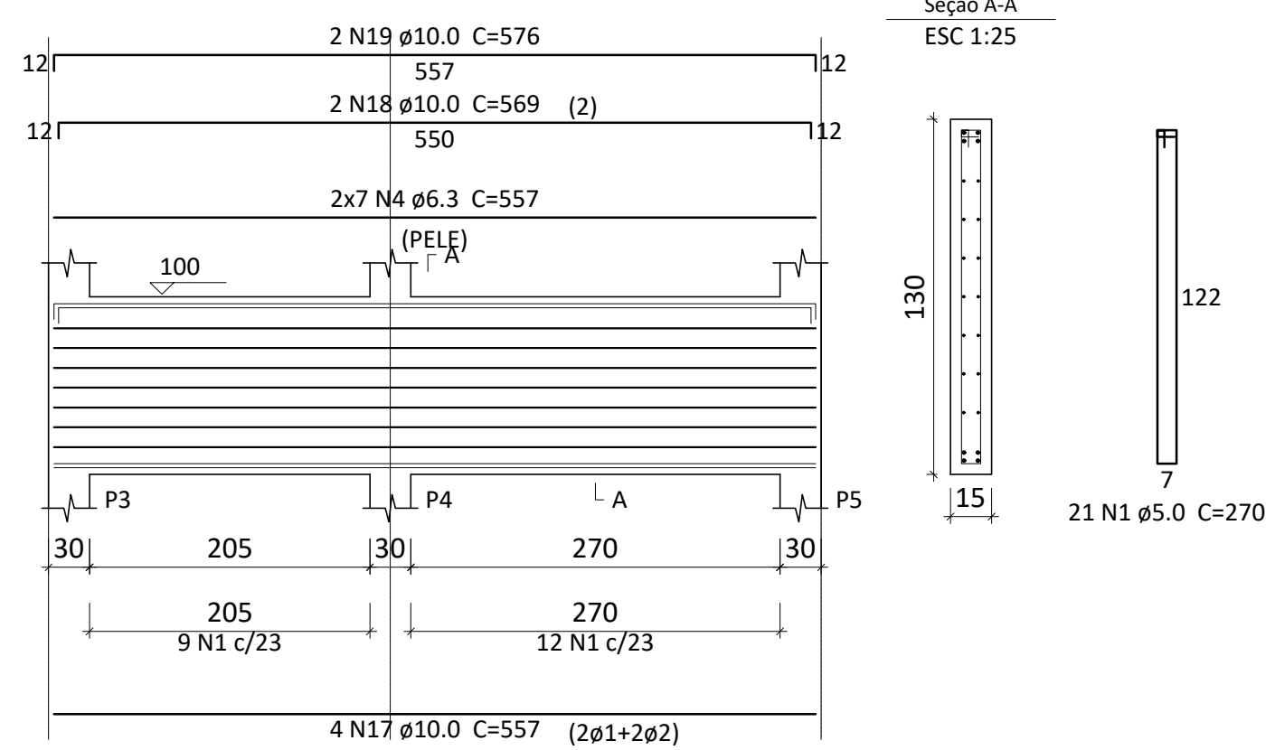
V2 ESC 1:50
