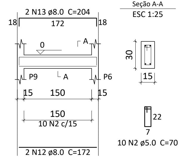
V9 ESC 1:50
