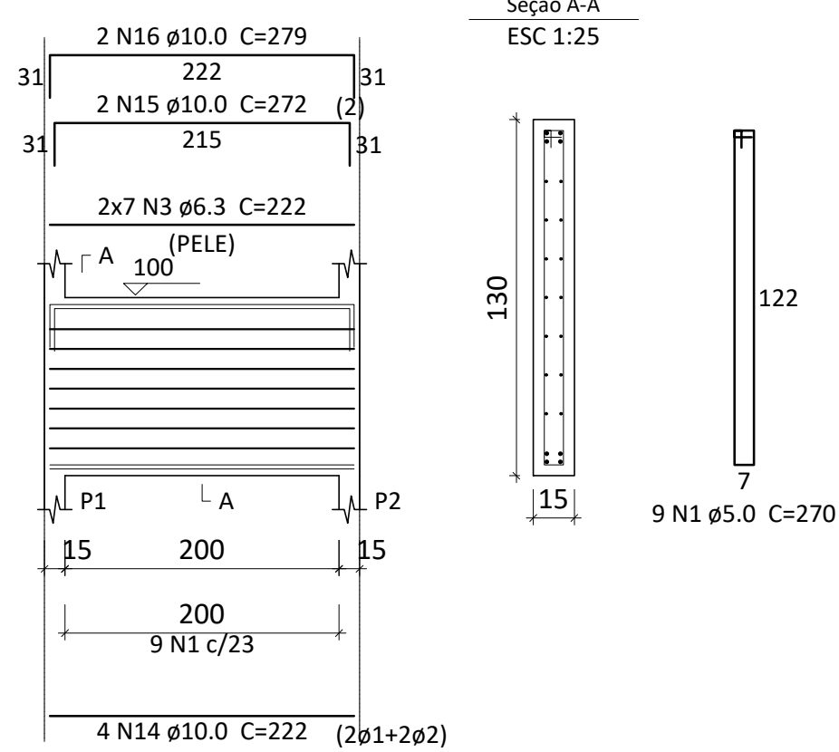
V1 ESC 1:50
