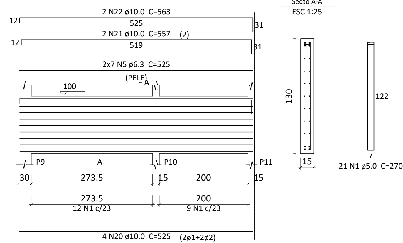
V4 ESC 1:50
