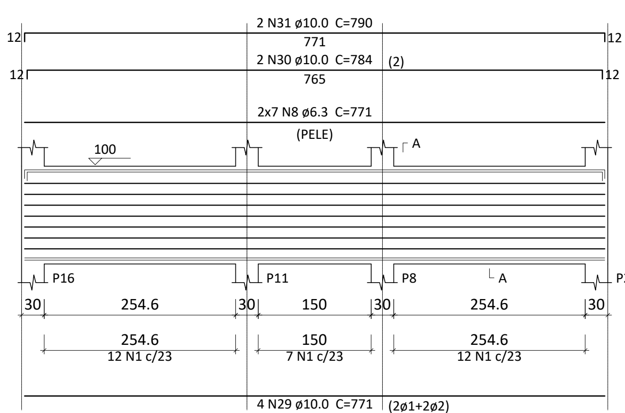
V12 ESC 1:50
