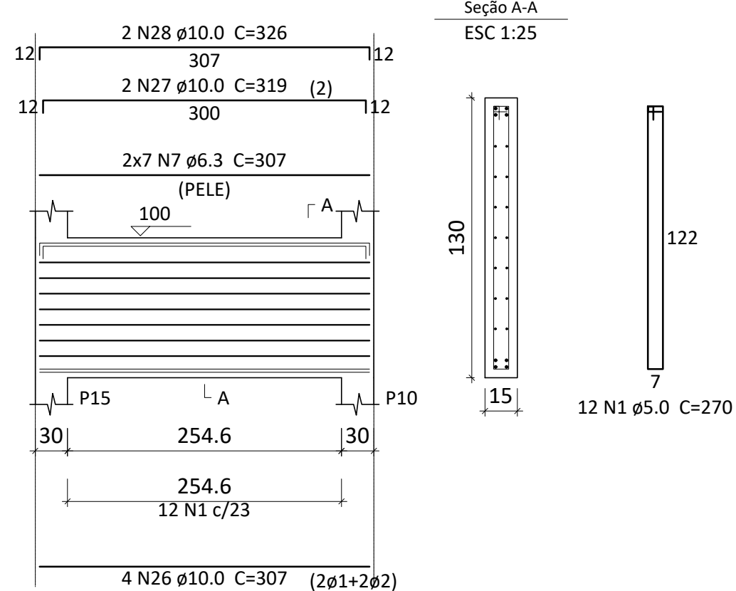
V10 ESC 1:50
