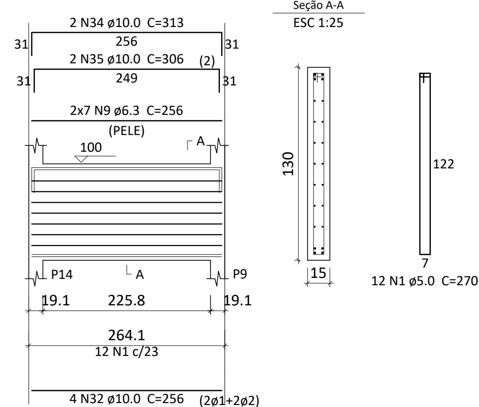
V14 ESC 1:50
