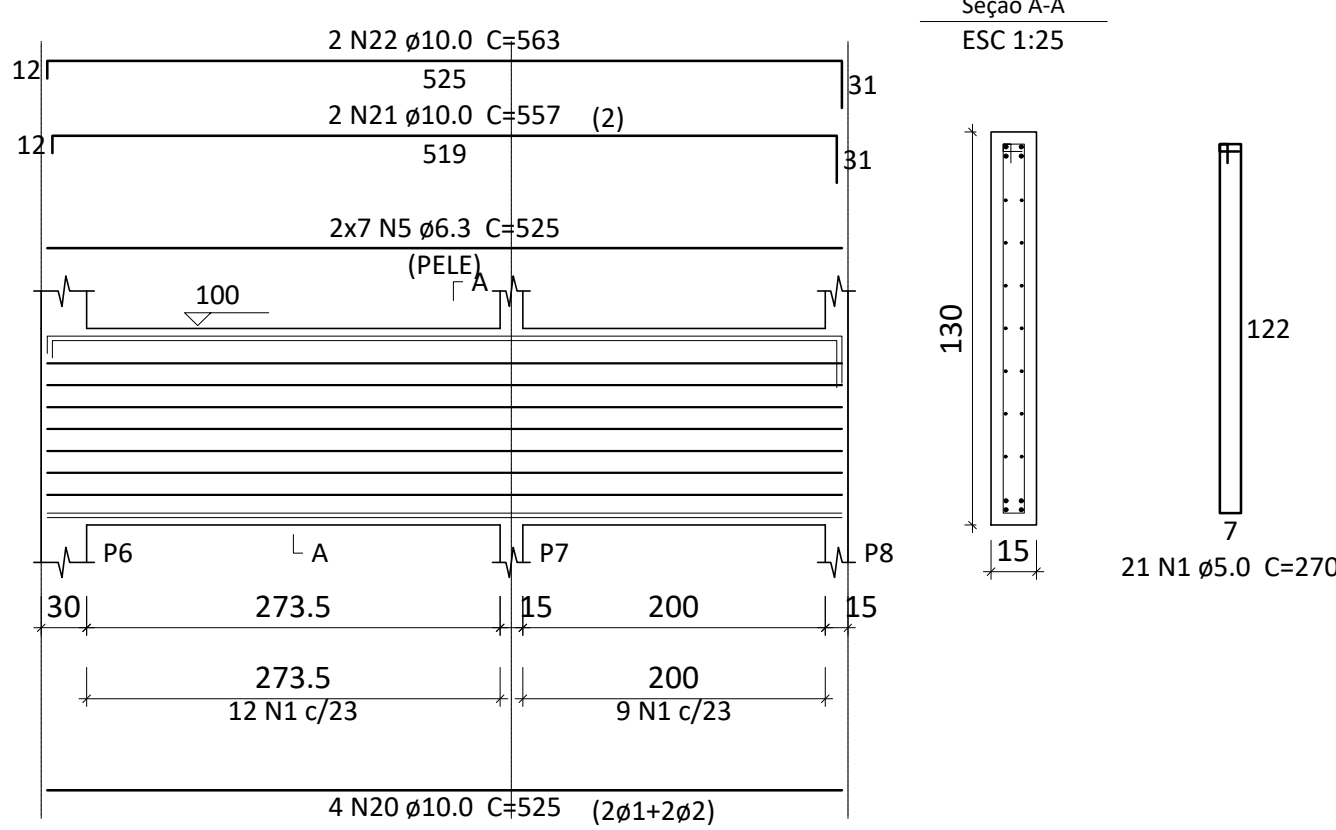
V3 ESC 1:50
