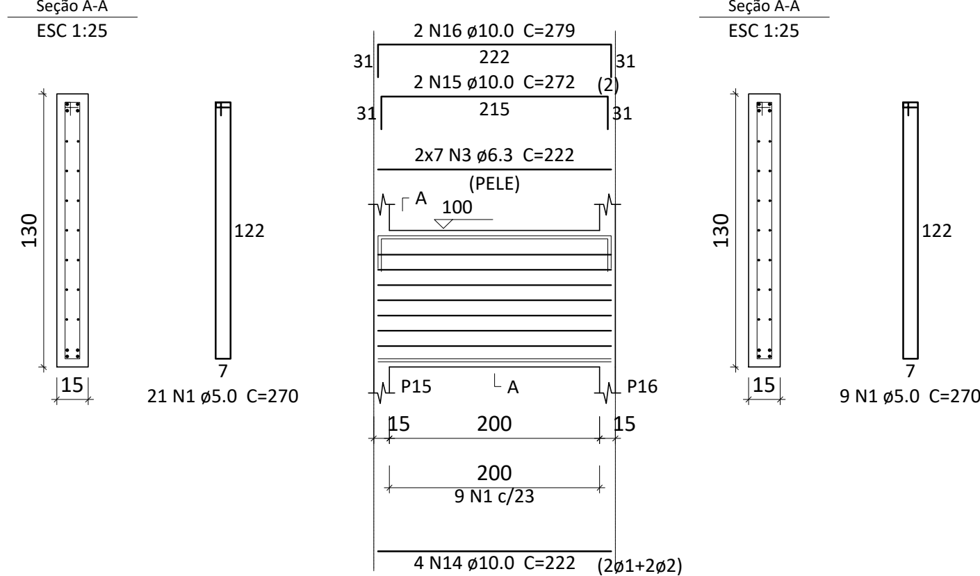
V6 ESC 1:50
