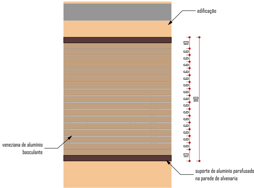
Detalhe 02 - Elevação - Veneziana de Alumínio ESC 1:20
