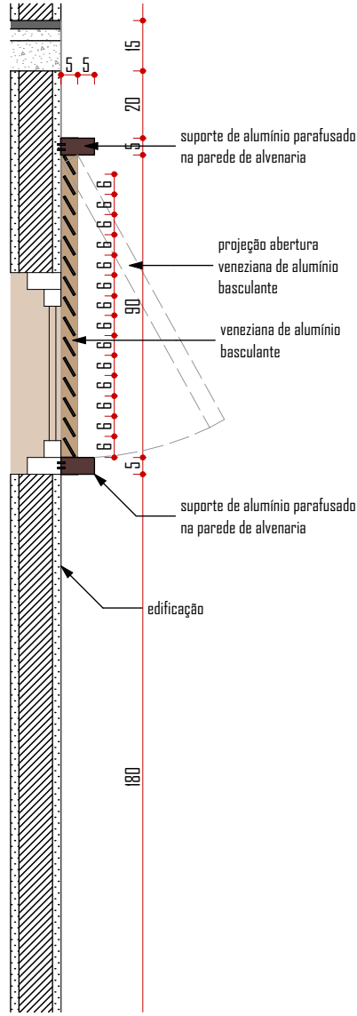
Detalhe 02 - Corte - Veneziana de Alumínio ESC 1:20
