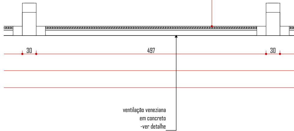
Detalhe 03 - Planta Baixa - Veneziana em Concreto ESC 1:50
