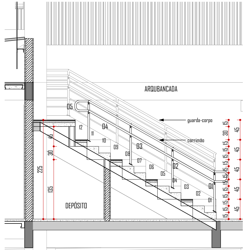
Detalhe 01- Corte - Arquibancada ESC 1:50
