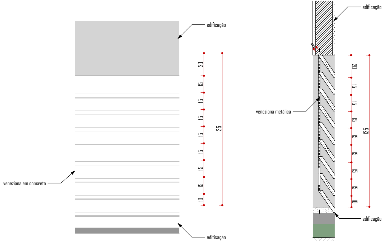
Detalhe 03 - Elevação - Veneziana em Concreto ESC 1:20
