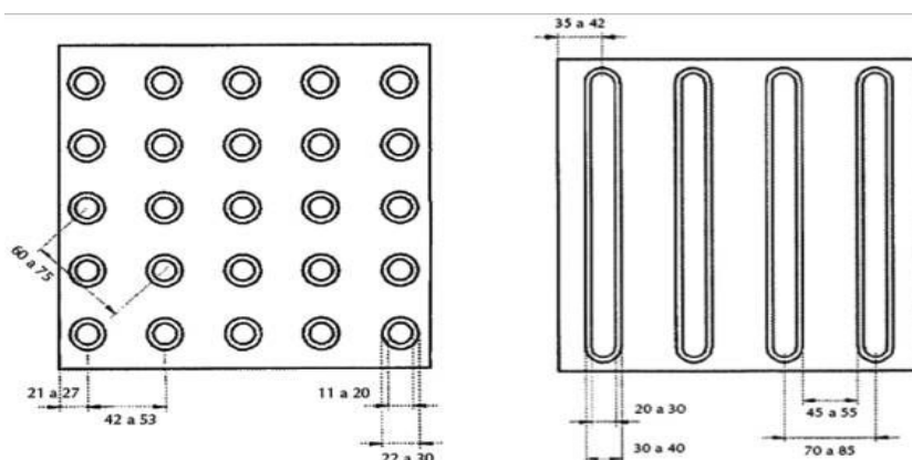
Figura 1 – Imagem representativa de instalação de piso podotátil guia em paver
