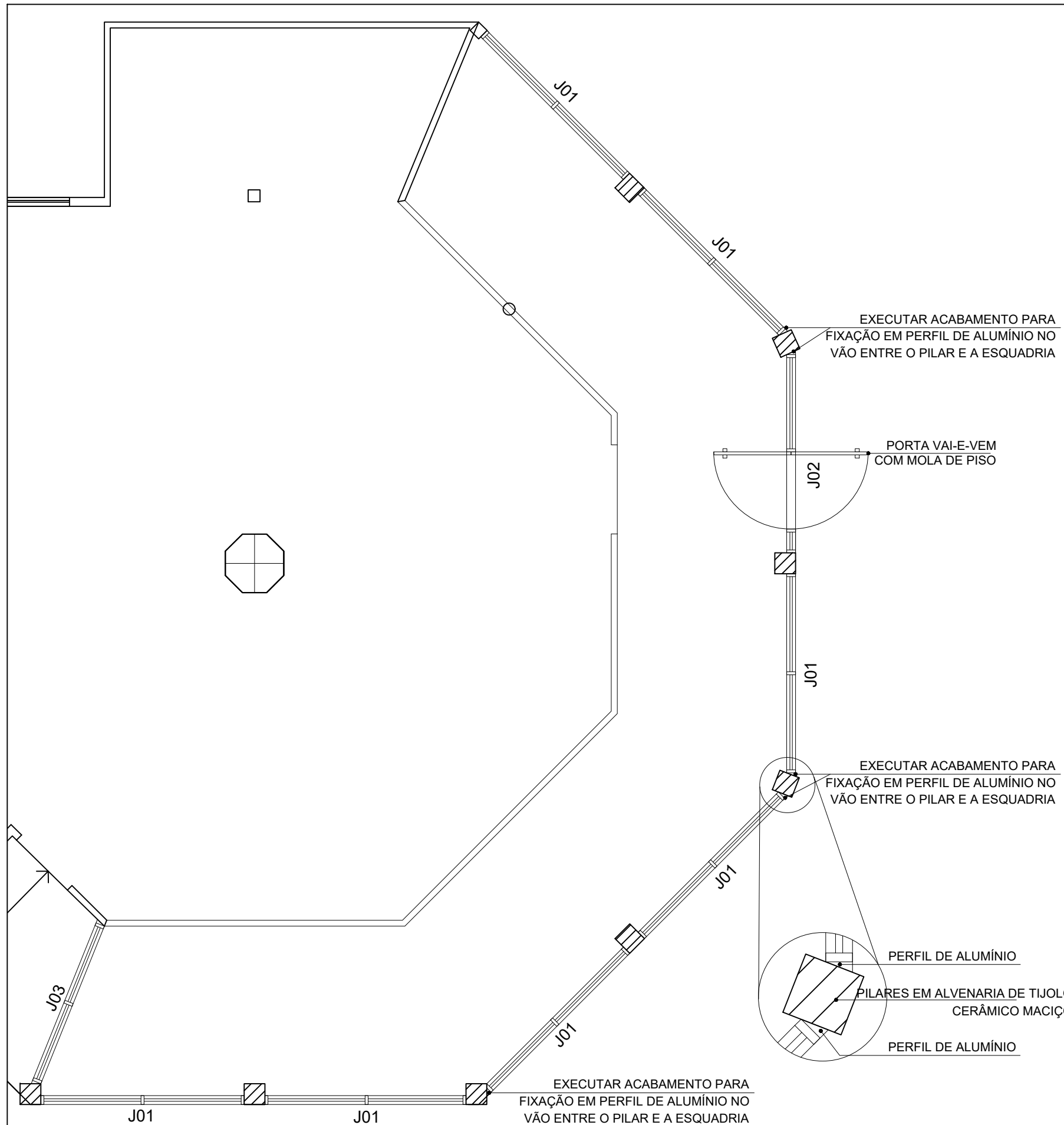
PLANTA BAIXA ESQUADRIAS ESC. 1/75
