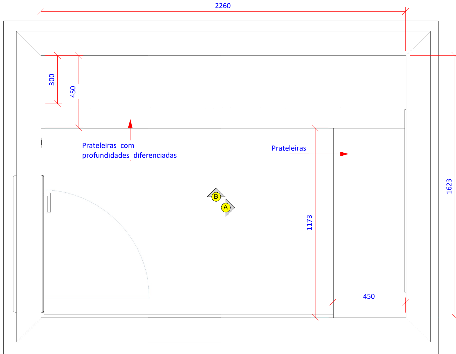
VISTA SUPERIOR
