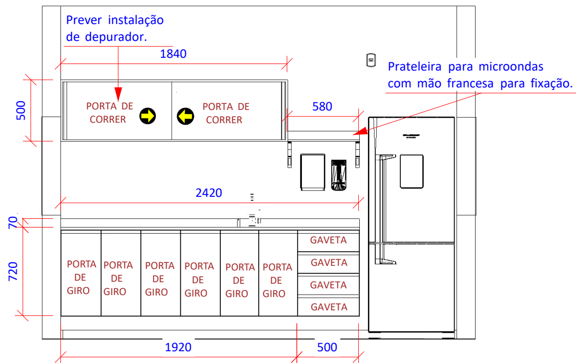
VISTA A - EXTERNO
