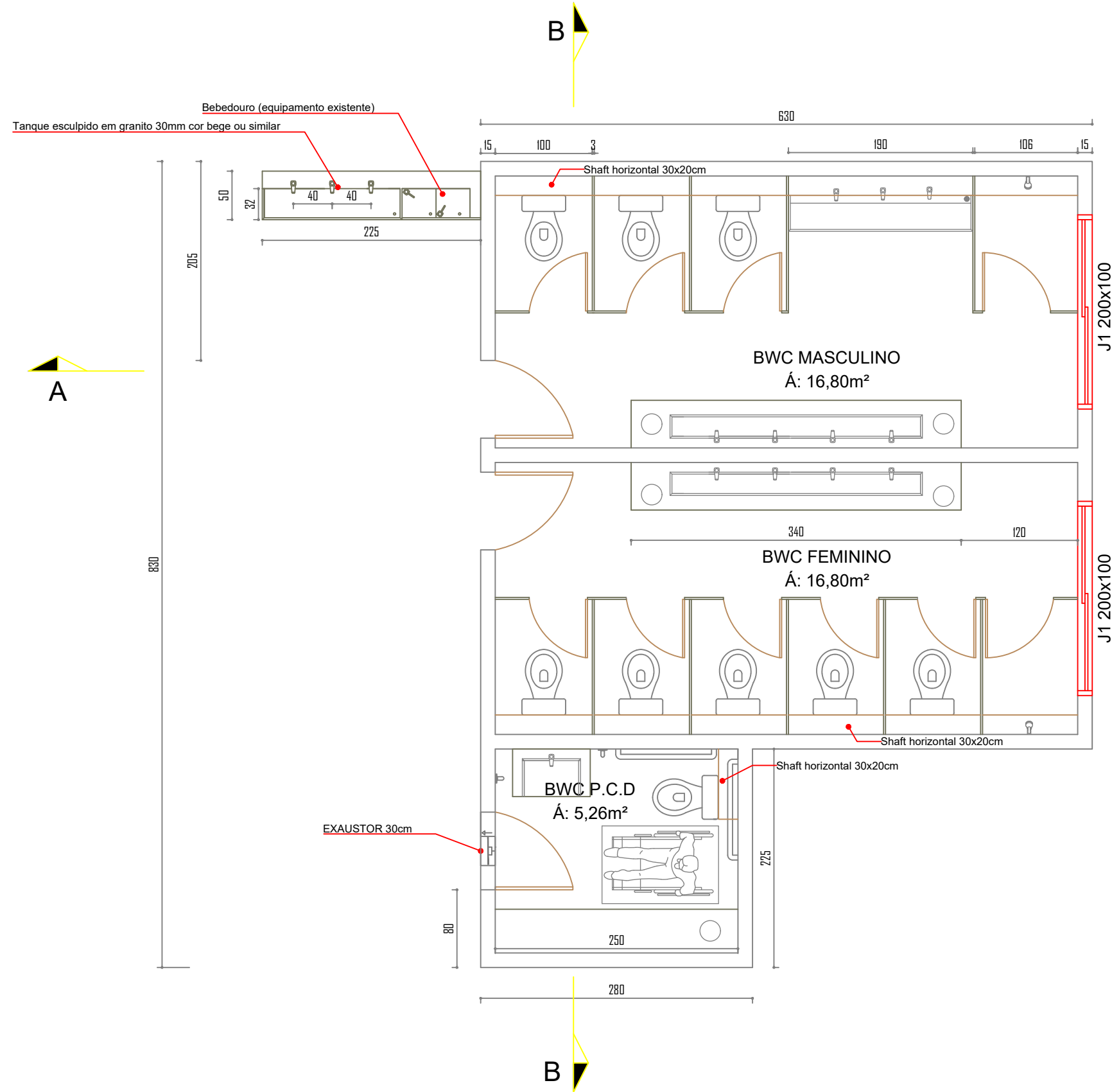
PLANTA BAIXA - SANITÁRIOS ESC: 1/50 ÁREA: 44,41m²
