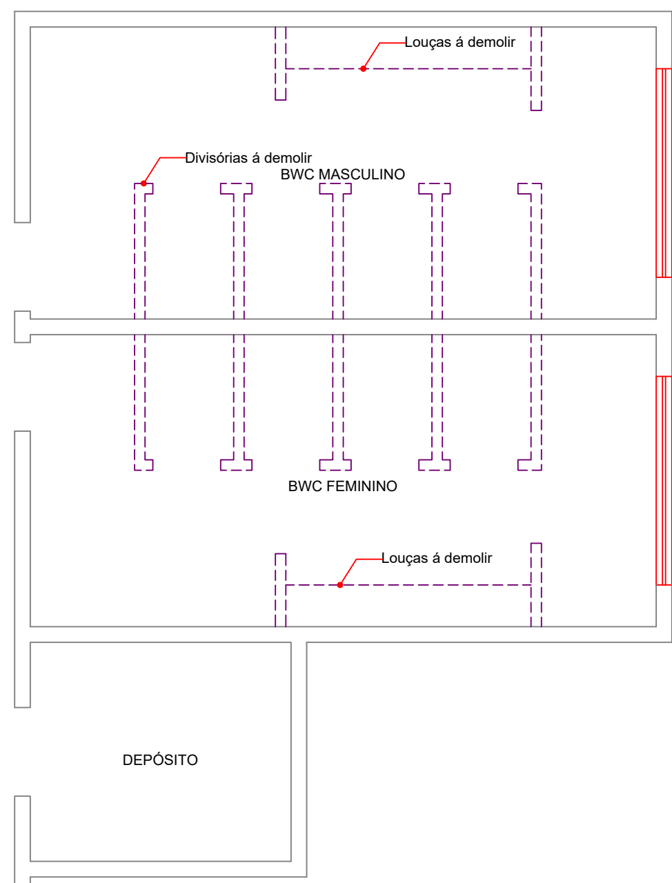
PLANTA DE REMOÇÕES ESC: 1/50 ÁREA: 44,41m²
