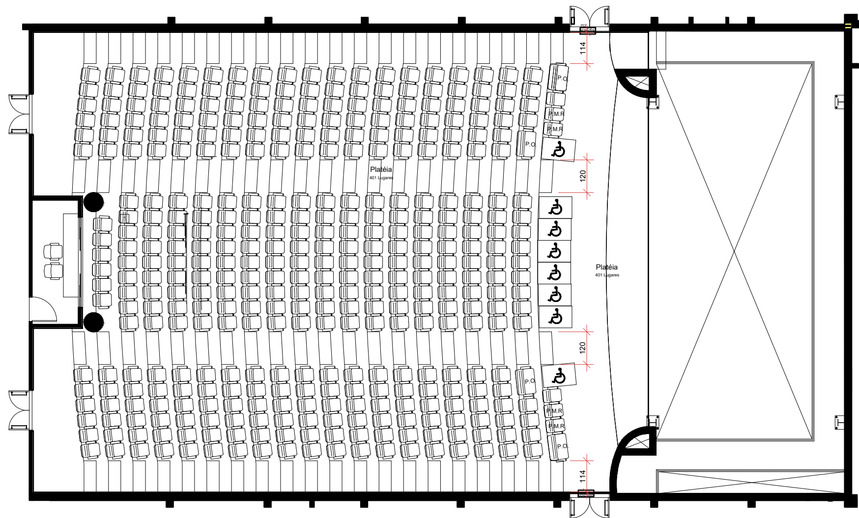
1 PLANTA DISPOSIÇÃO DE LUGARES Escala 1/125
