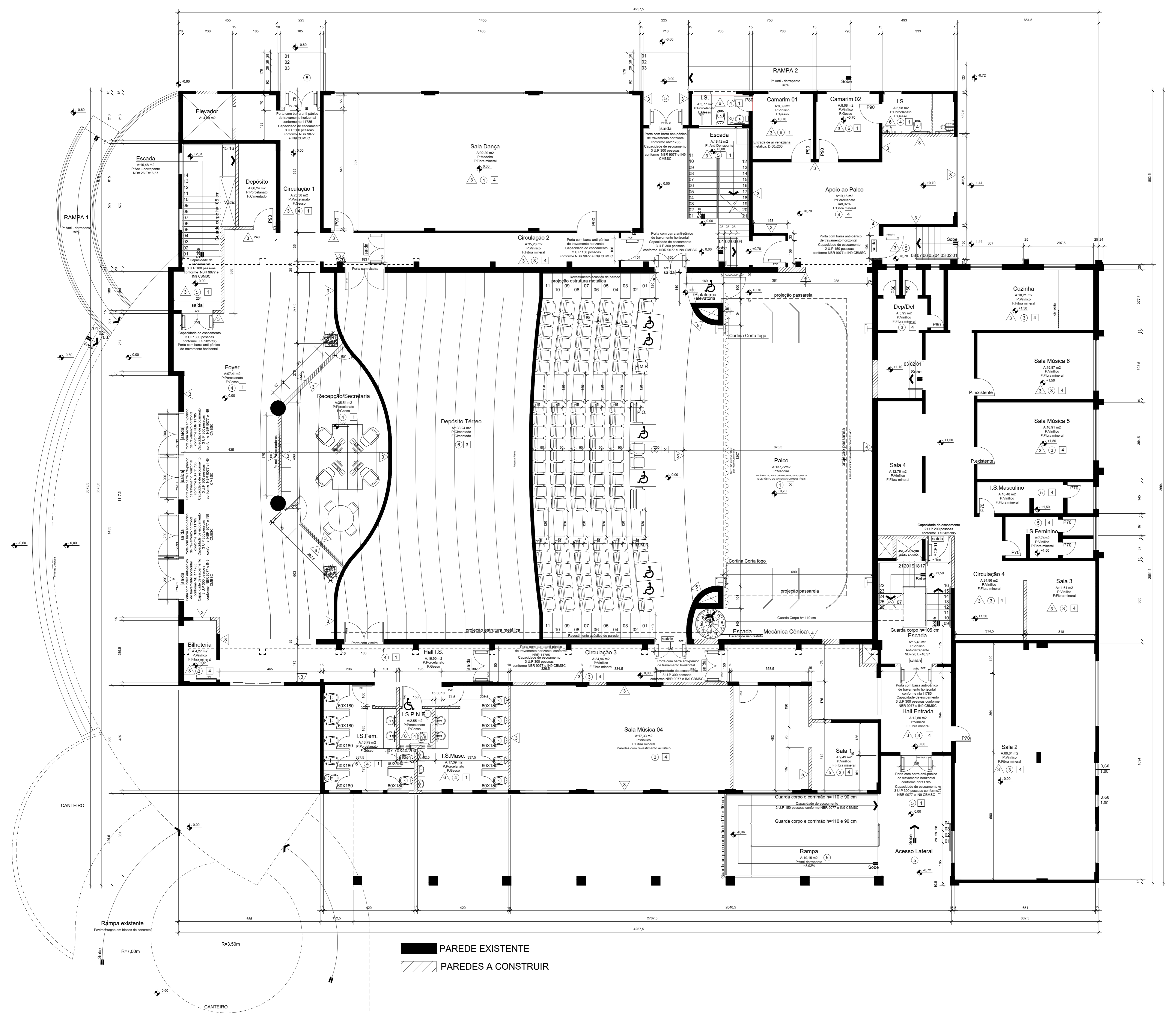
1 PLANTA BAIXA 1º PAVIMENTO Escala 1/75
