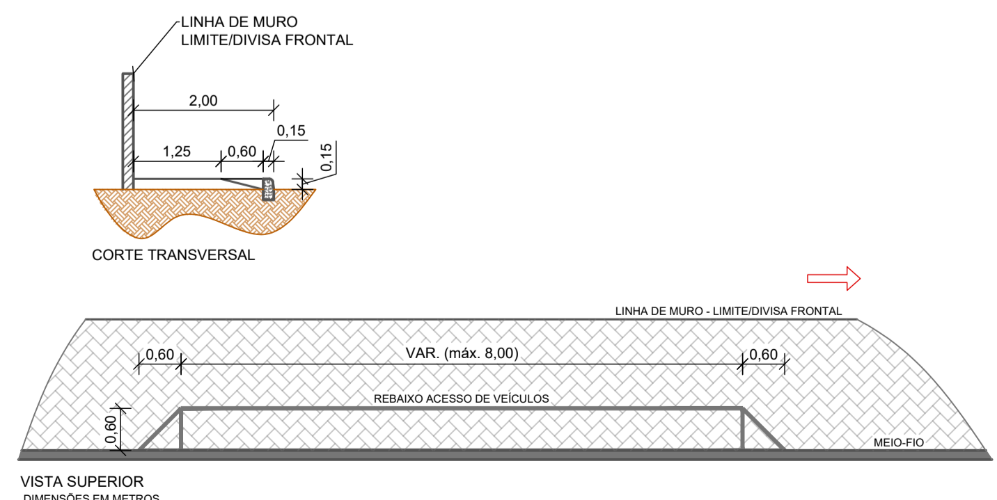
4 DETALHE PASSEIO REBAIXO ACESSO DE VEÍCULOS ESCALA: 1:75
