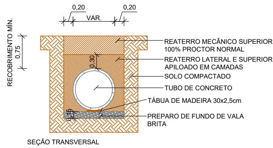
3 DETALHE VALA SISTEMA DRENAGEM ESCALA: 1/50
