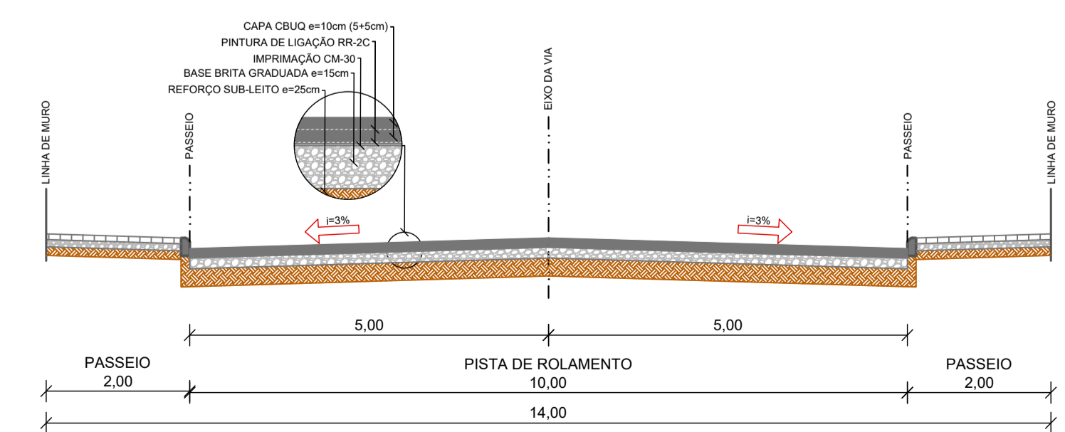
3 SEÇÃO TRANSVERSAL ESCALA: 1:75
