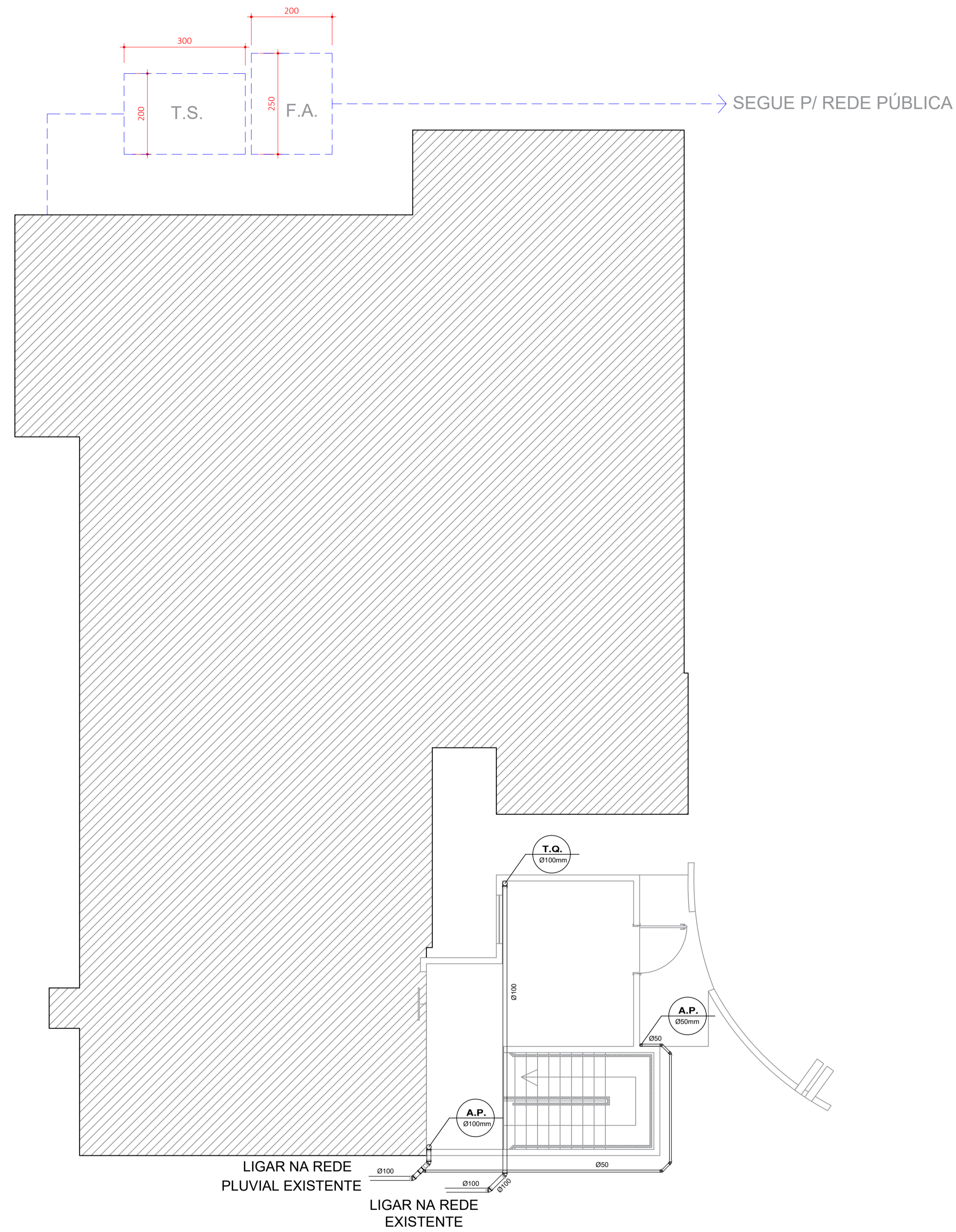
PLANTA BAIXA - TÉRREO PROJETO SANITÁRIO/ PLUVIAL ESCALA 1:75
