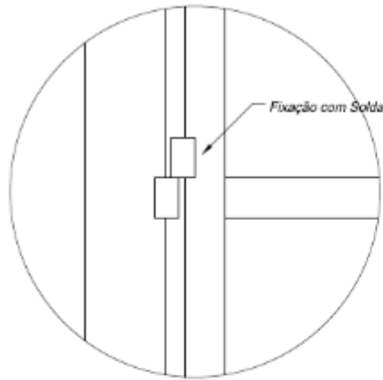
Detalhe Pino Gonzo 5/8
