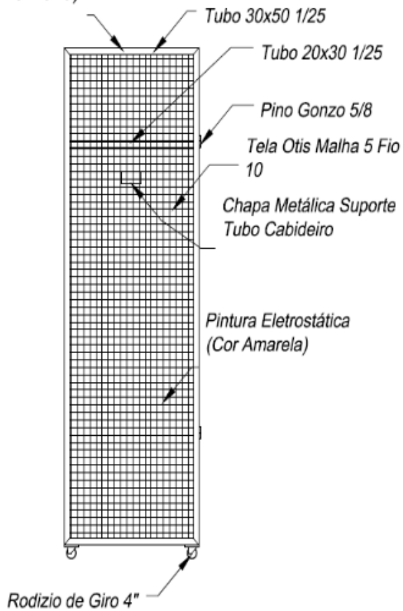
Vista Lateral
