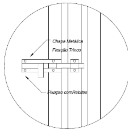
Detalhe Trinco Galvanizado
