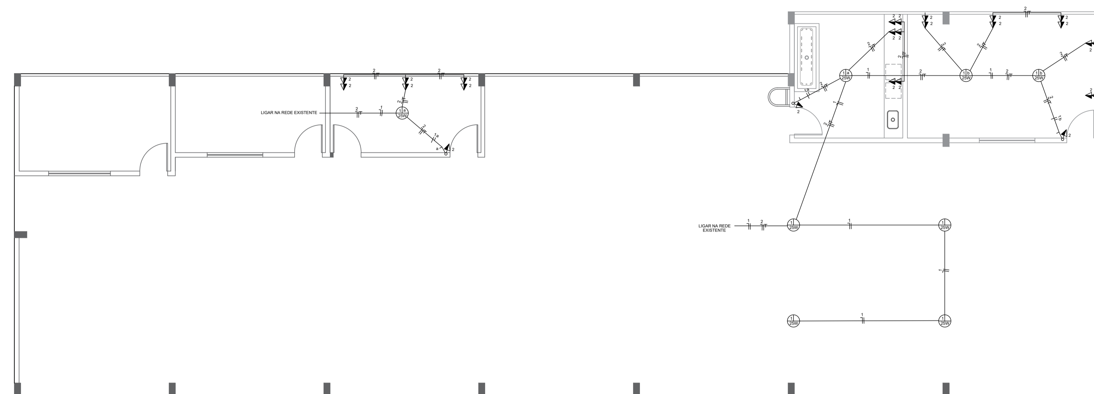
PLANTA BAIXA - TÉRREO PROJETO ELÉTRICO ESCALA 1:75
