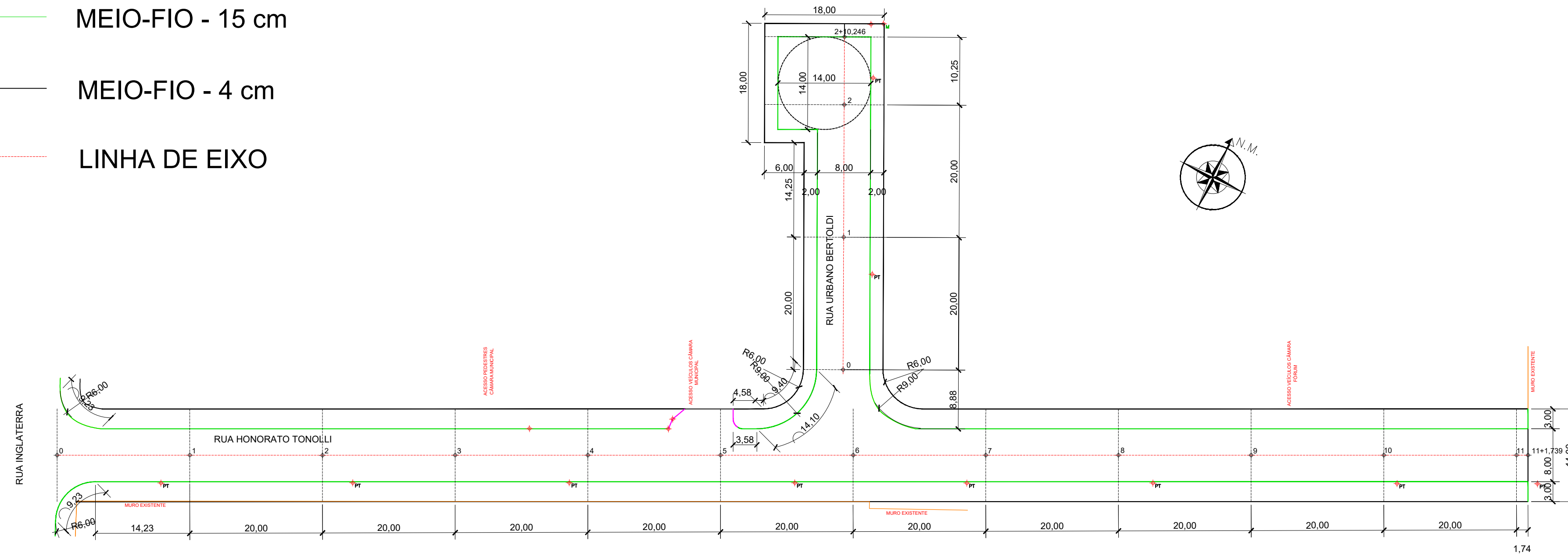
GEOMÉTRICO ESC: 1/500
