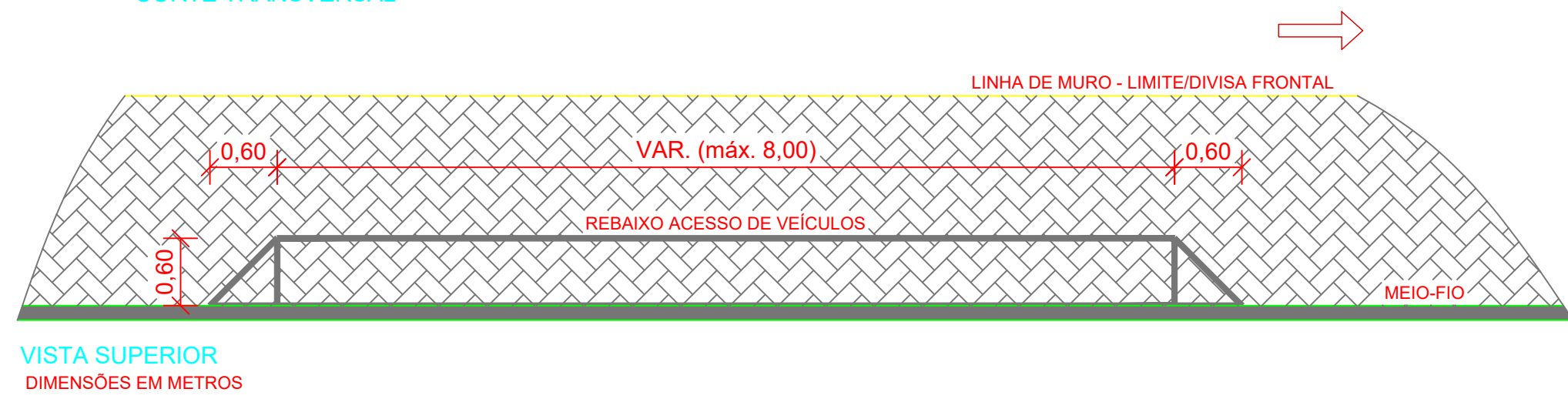
4 DETALHE PASSEIO REBAIXO ACESSO DE VEÍCULOS ESCALA: 1/75
