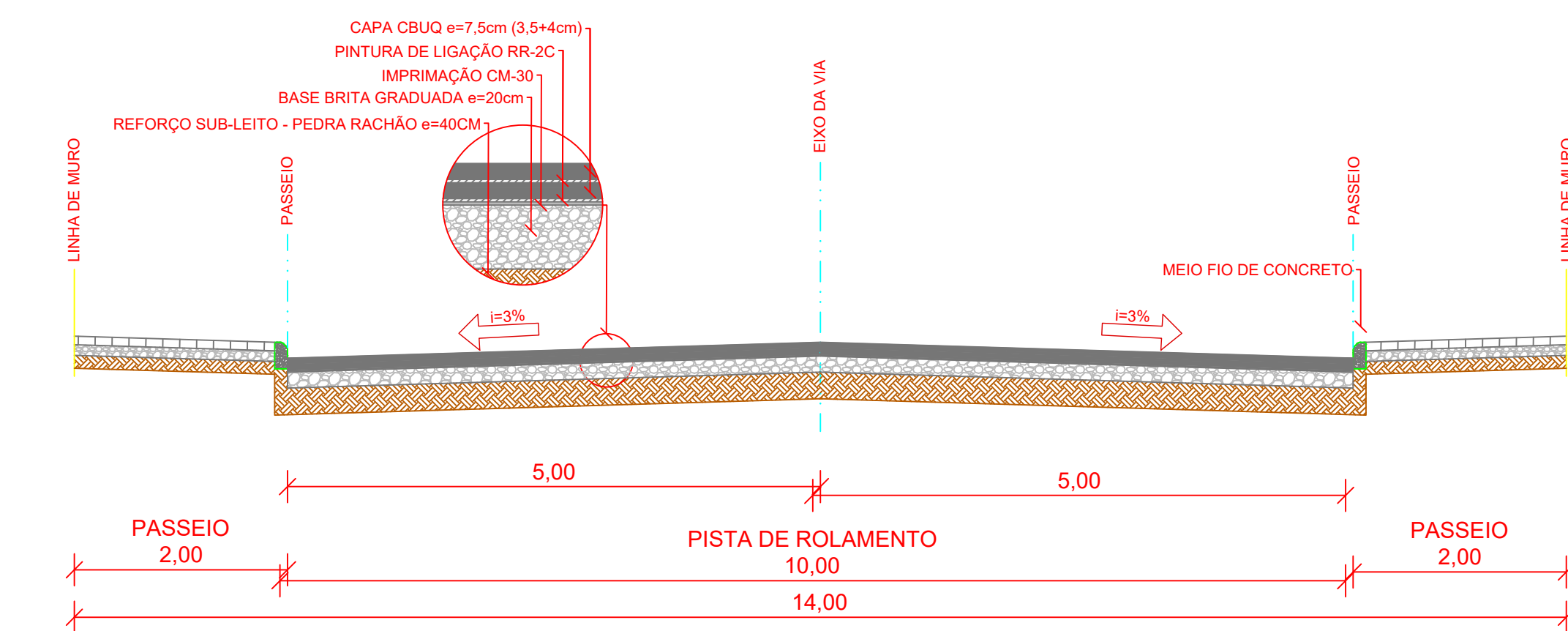
3 SEÇÃO TRANSVERSAL ESCALA: 1/75
