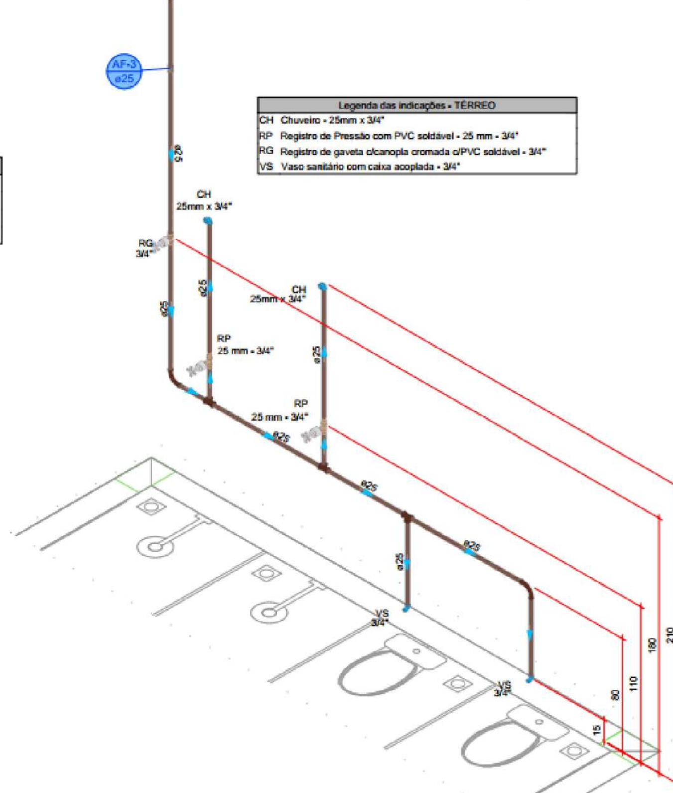
DETALHE HID-3 1:25
