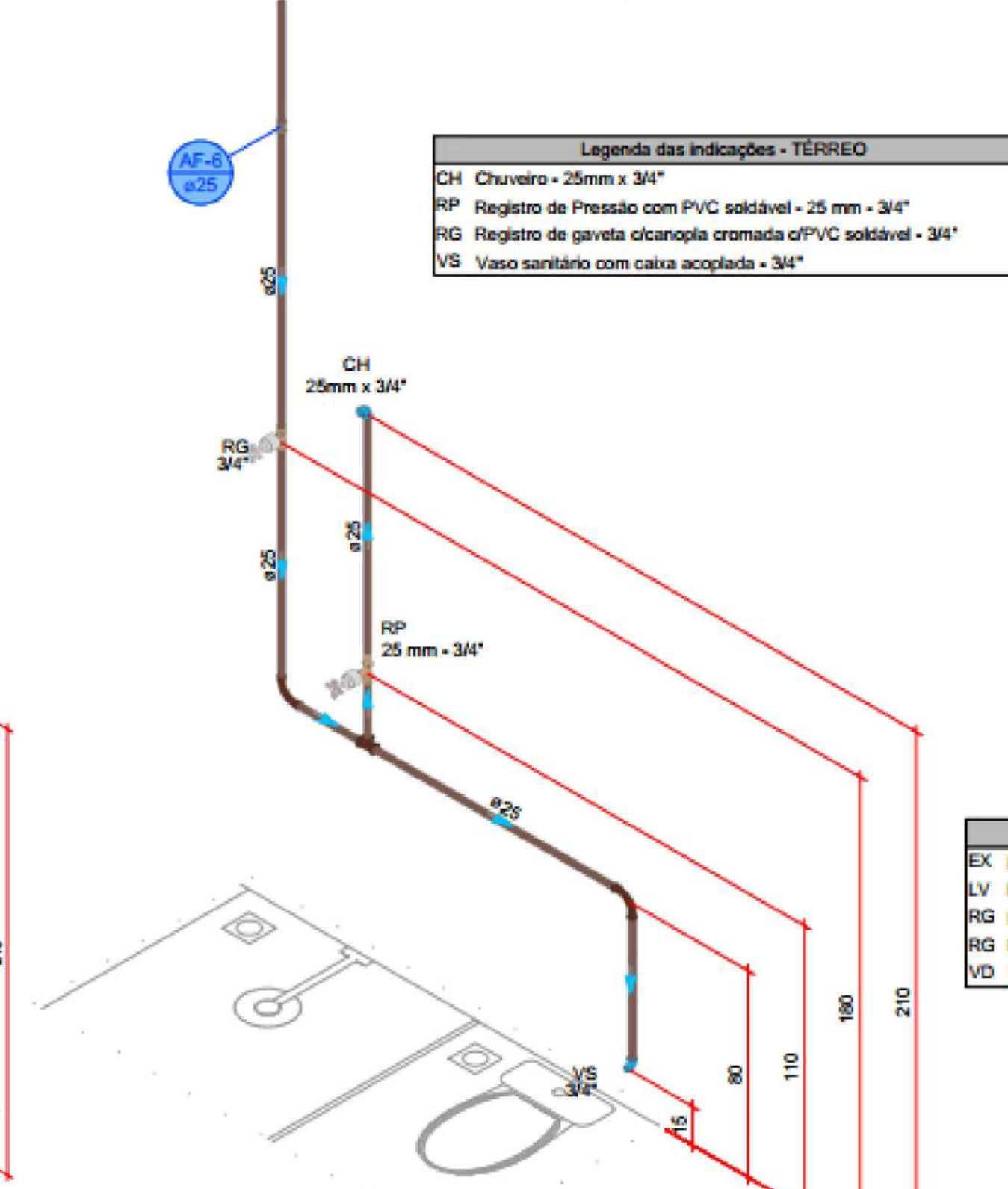
DETALHE HID-4 1:25
