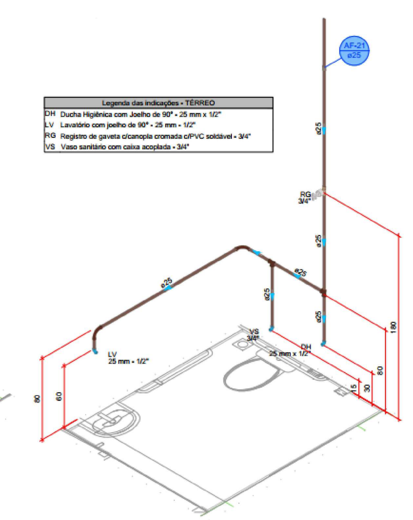
DETALHE HID-19 1:25
