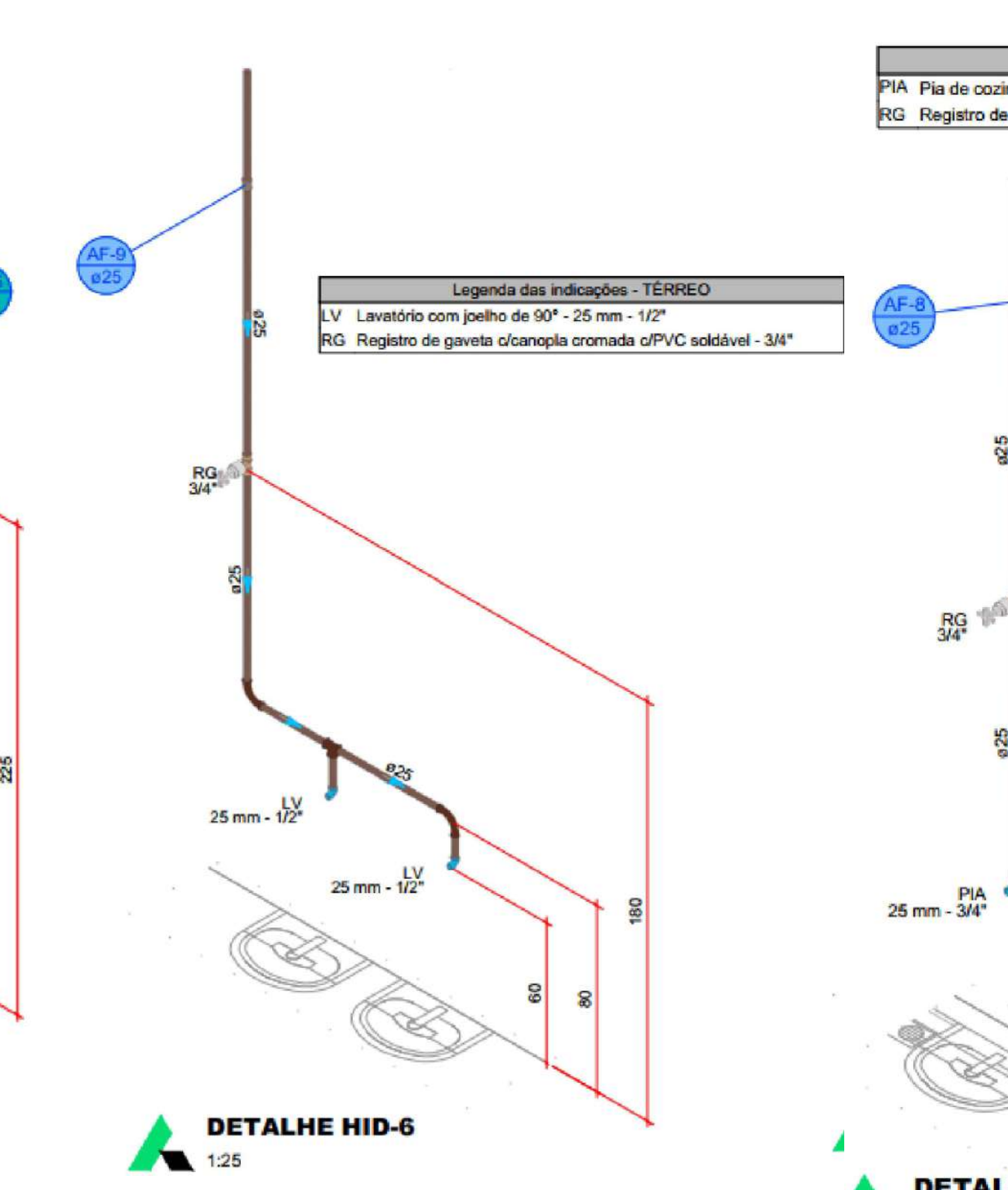
DETALHE HID-6 1:25
