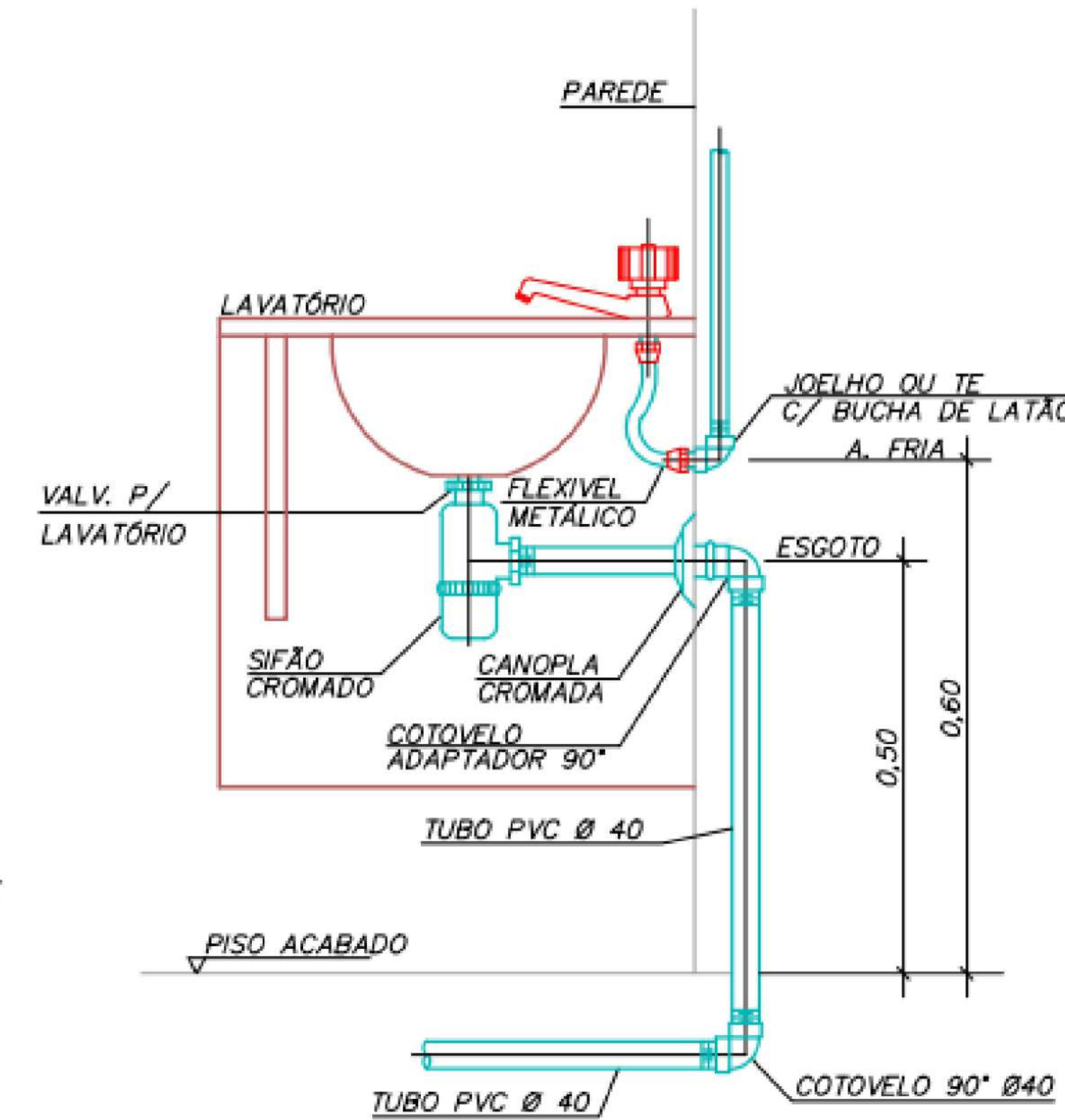
DETALHE LIGAÇÃO DE LAVATÓRIO SEM ESCALA
