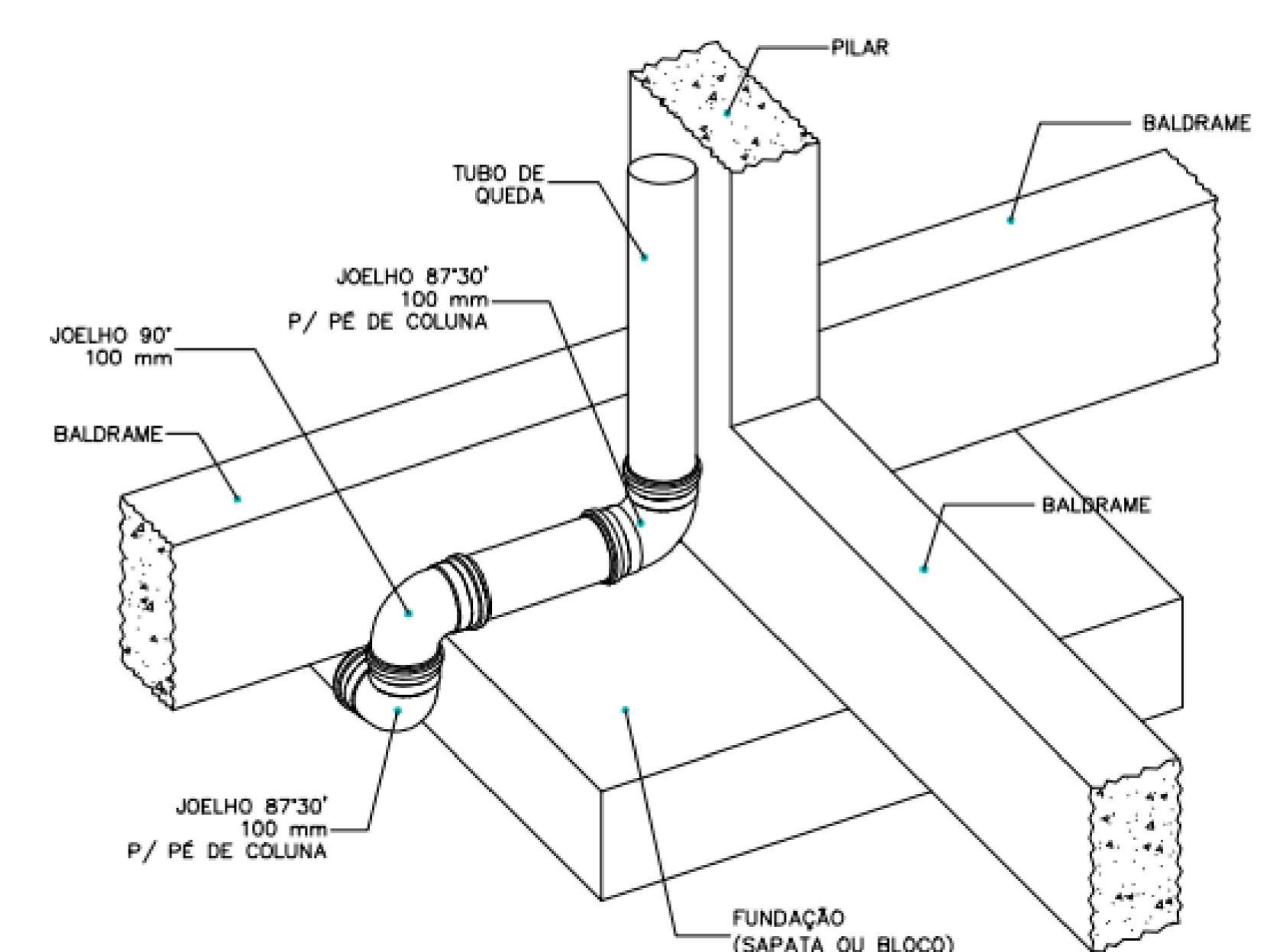
DETALHE DESVIO DE FUNDAÇÃO Sem Escala
