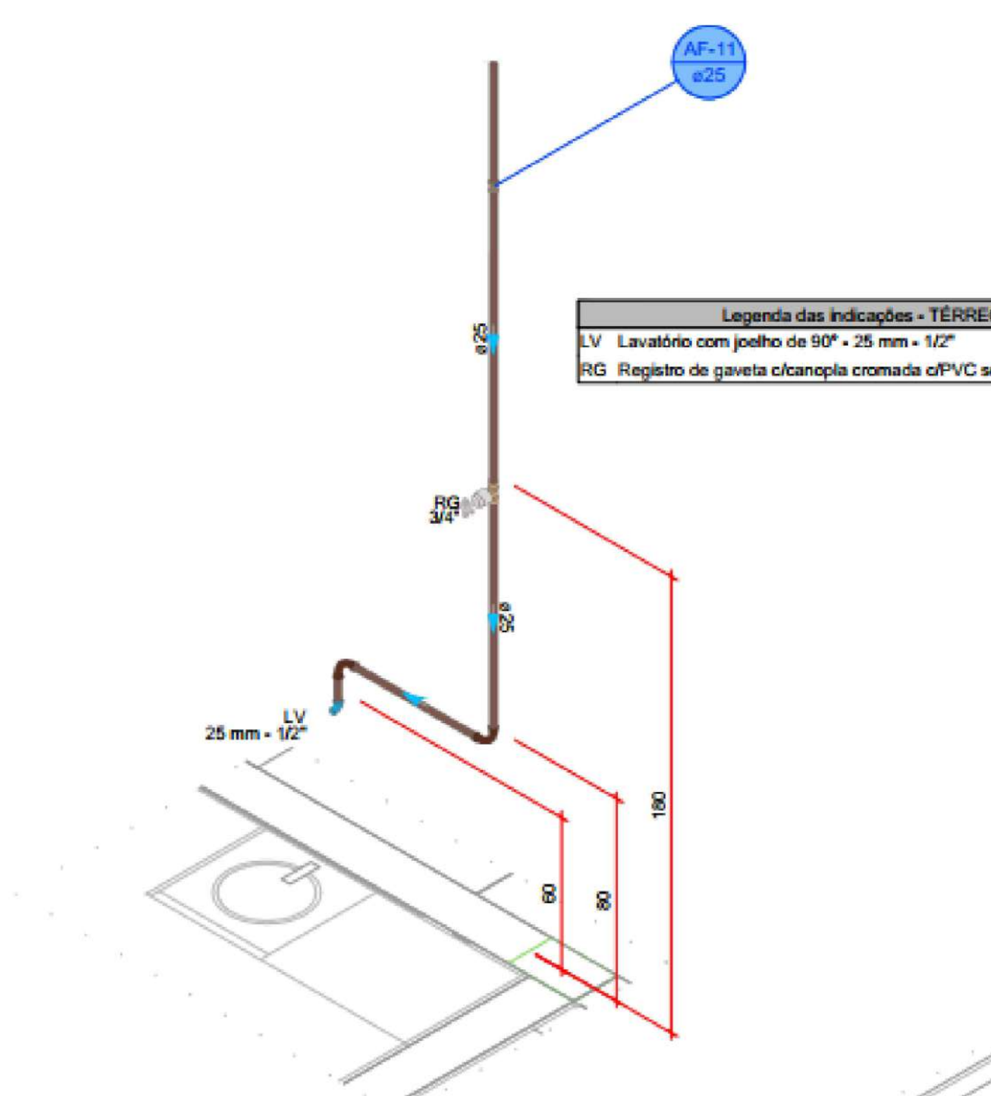
DETALHE HID-10 1:25
