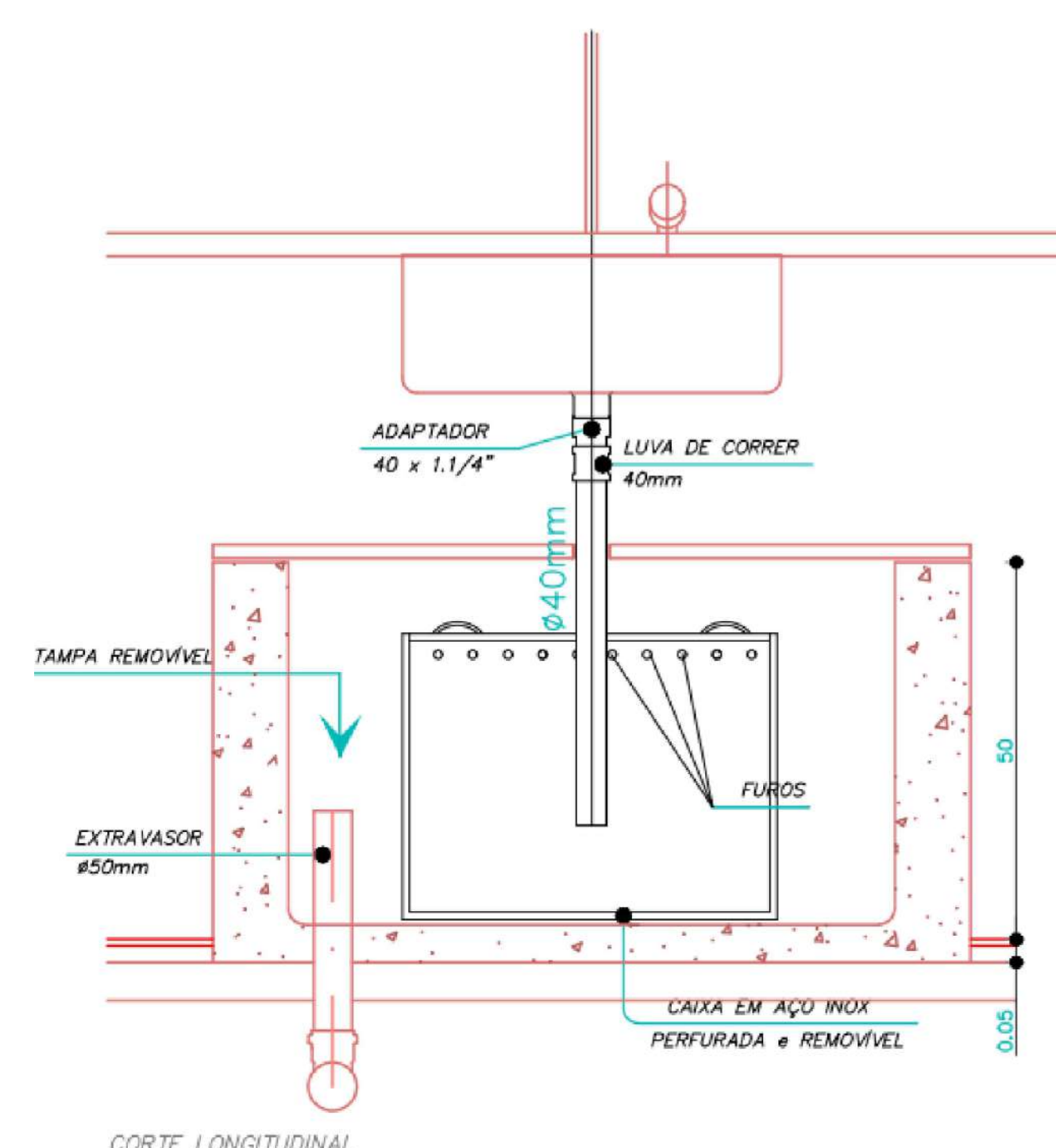
CORTE LONGITUDINAL
