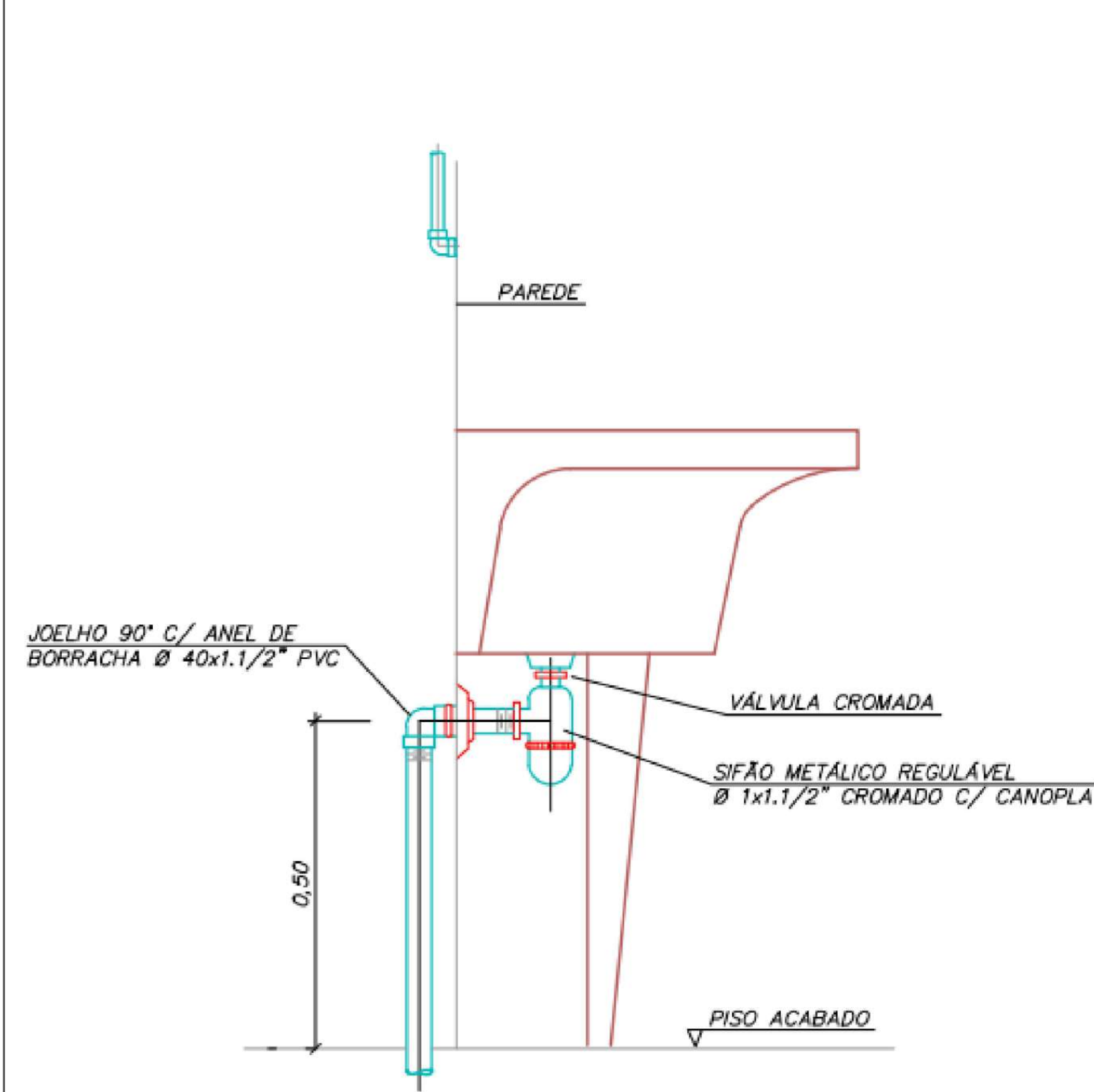
DETALHE LIGAÇÃO DE TANQUE SEM ESCALA
