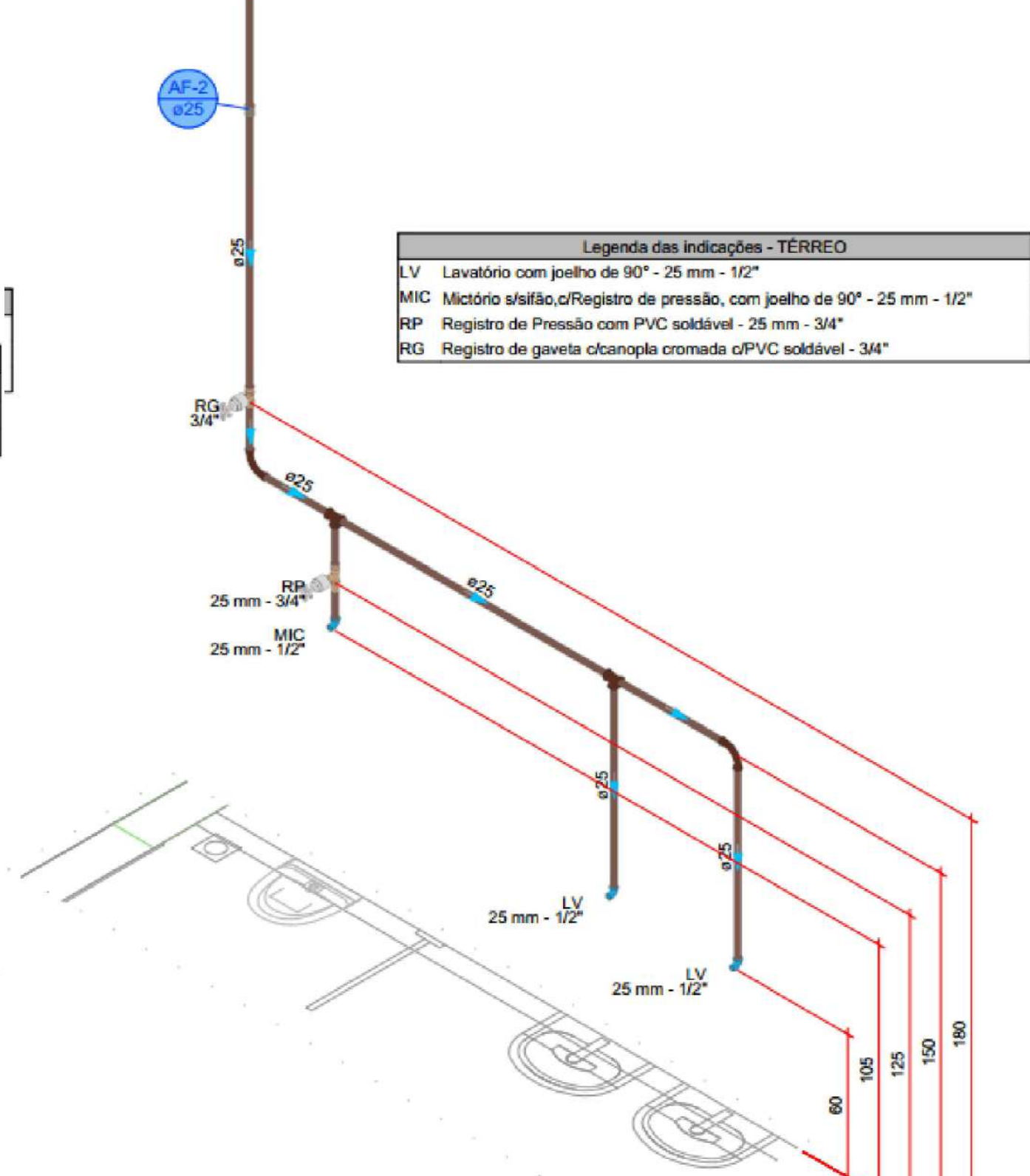
DETALHE HID-2 1:25
