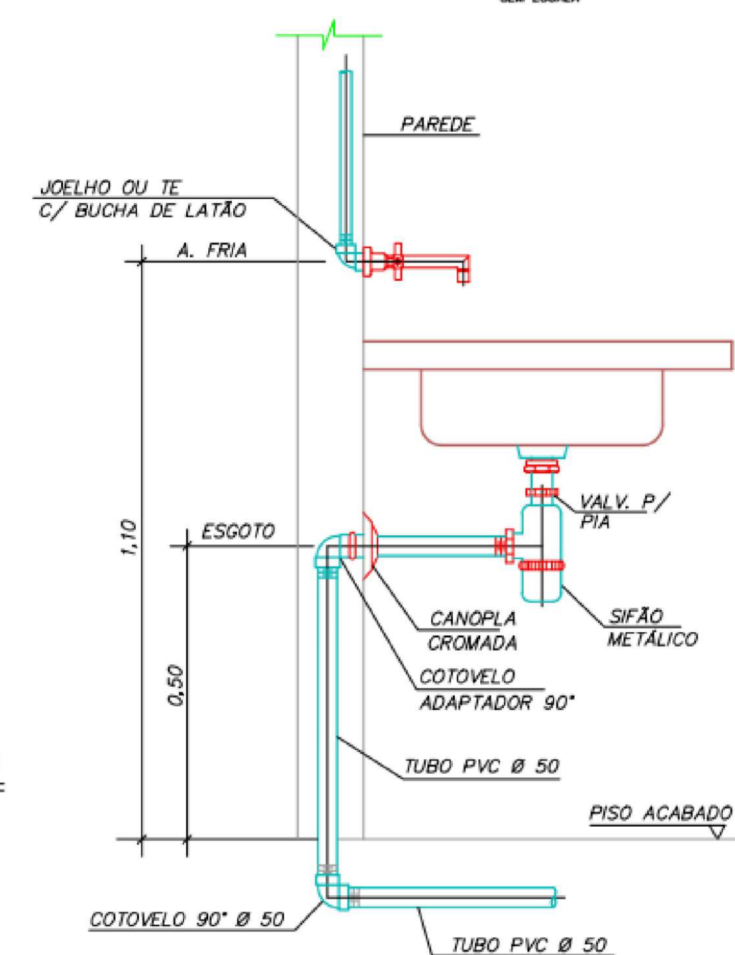
DETALHE DE LIGAÇÃO DE PIA SEM ESCALA
