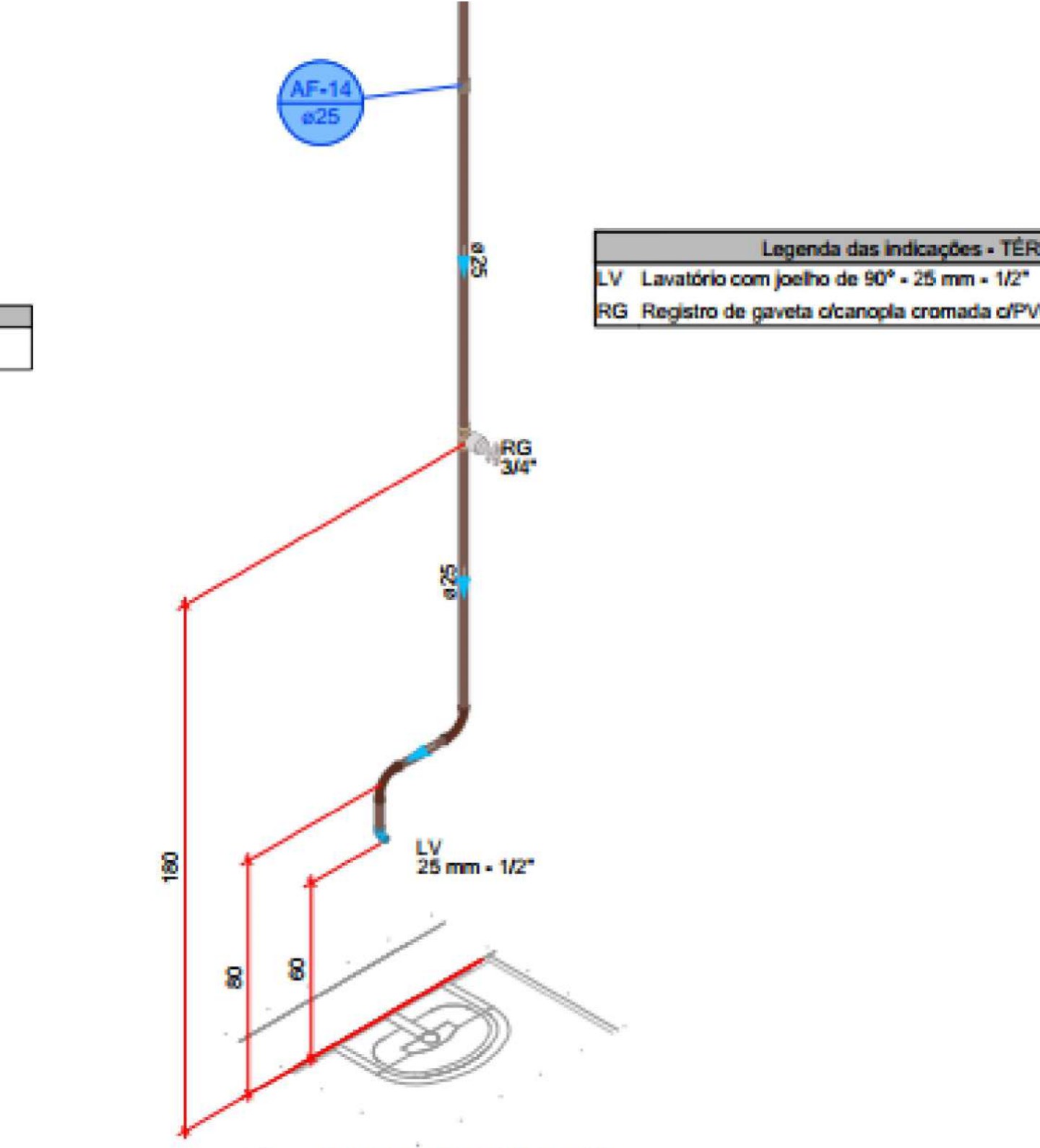
DETALHE HID-13 1:25
