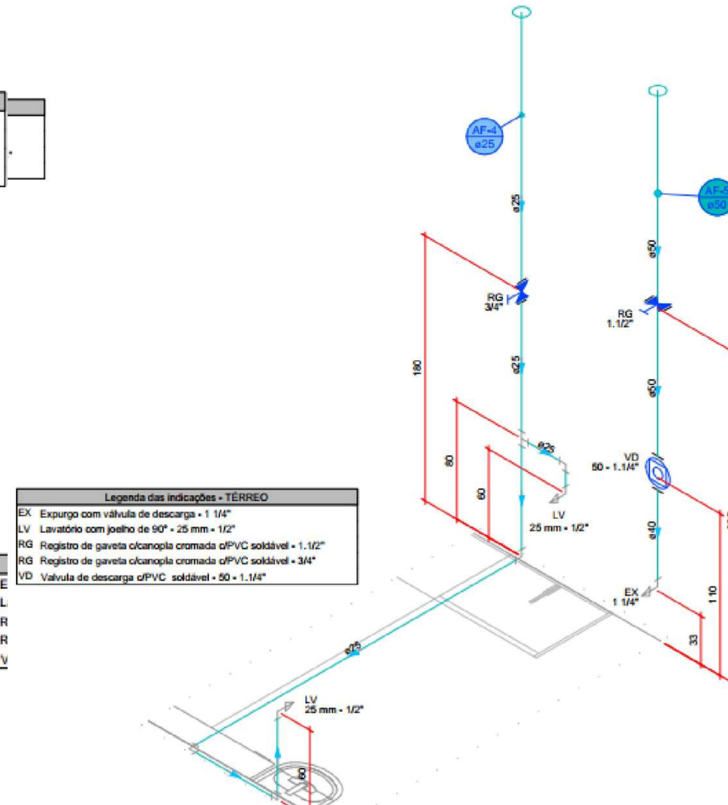
DETALHE HID-5 1:25
