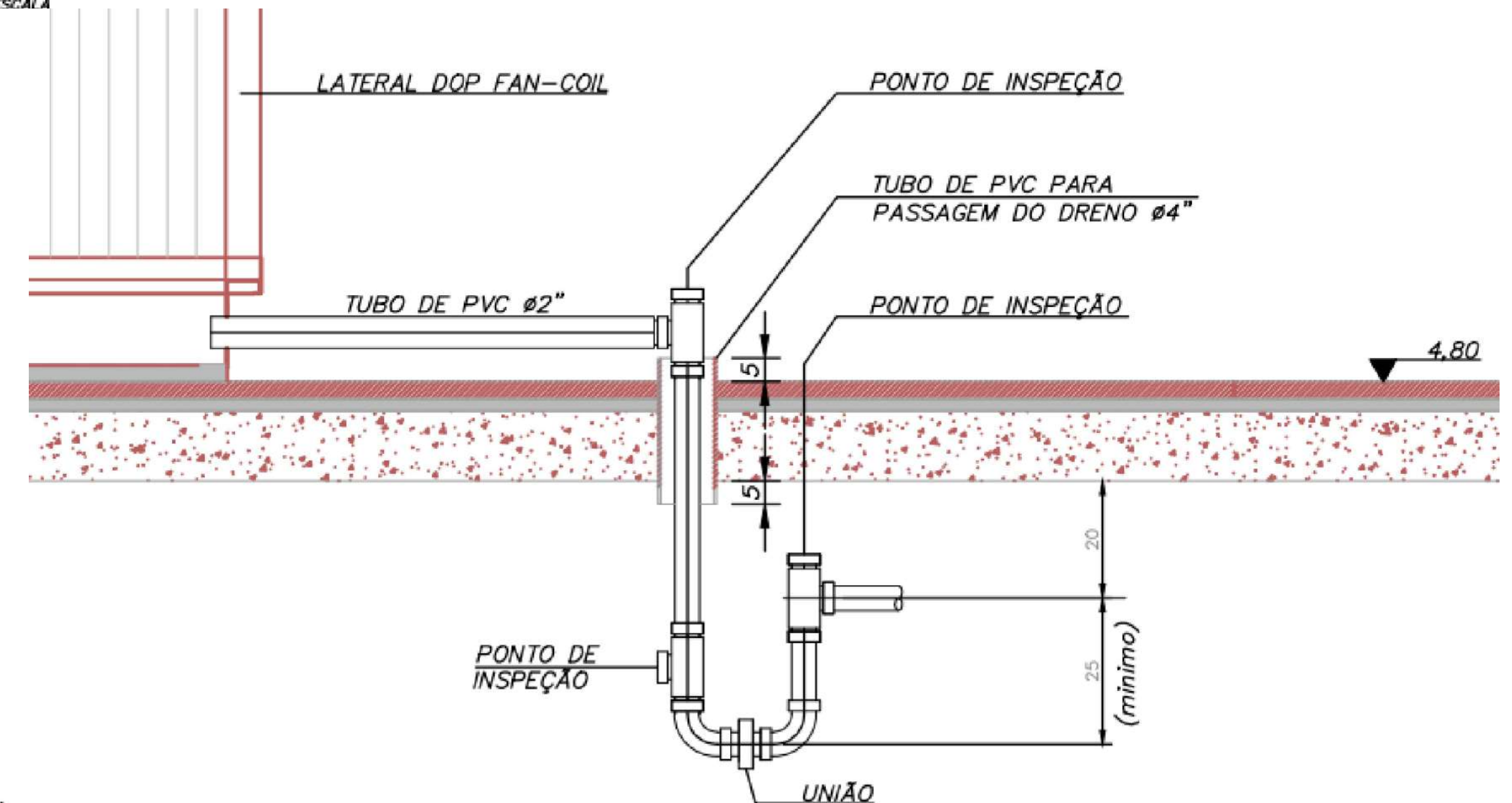
DETALHE DO SIFÃO P/ DRENO DO FAN COIL SEM ESCALA
