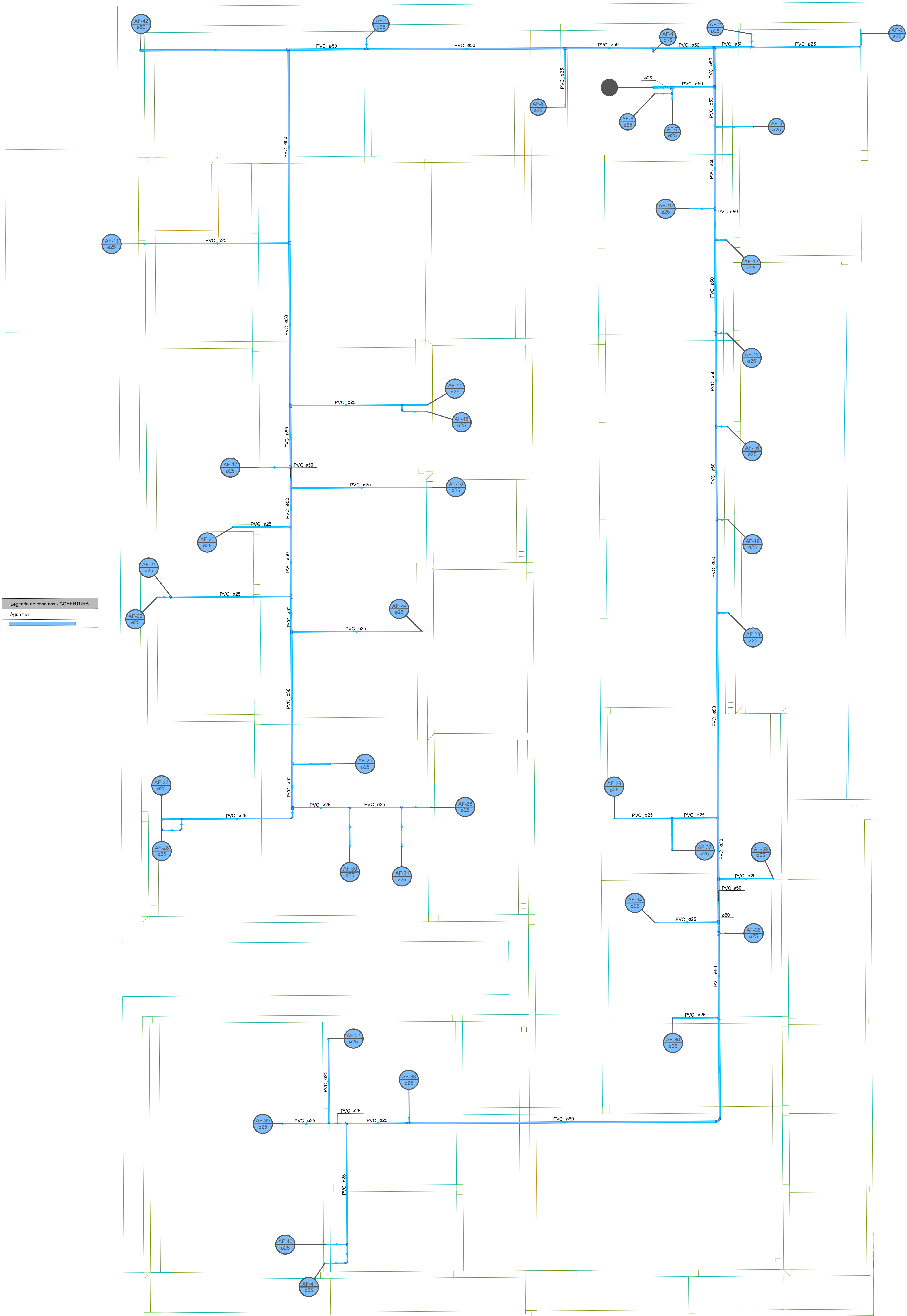
1 PLANTA BAIXA - COBERTURA - ÁGUA FRIA
