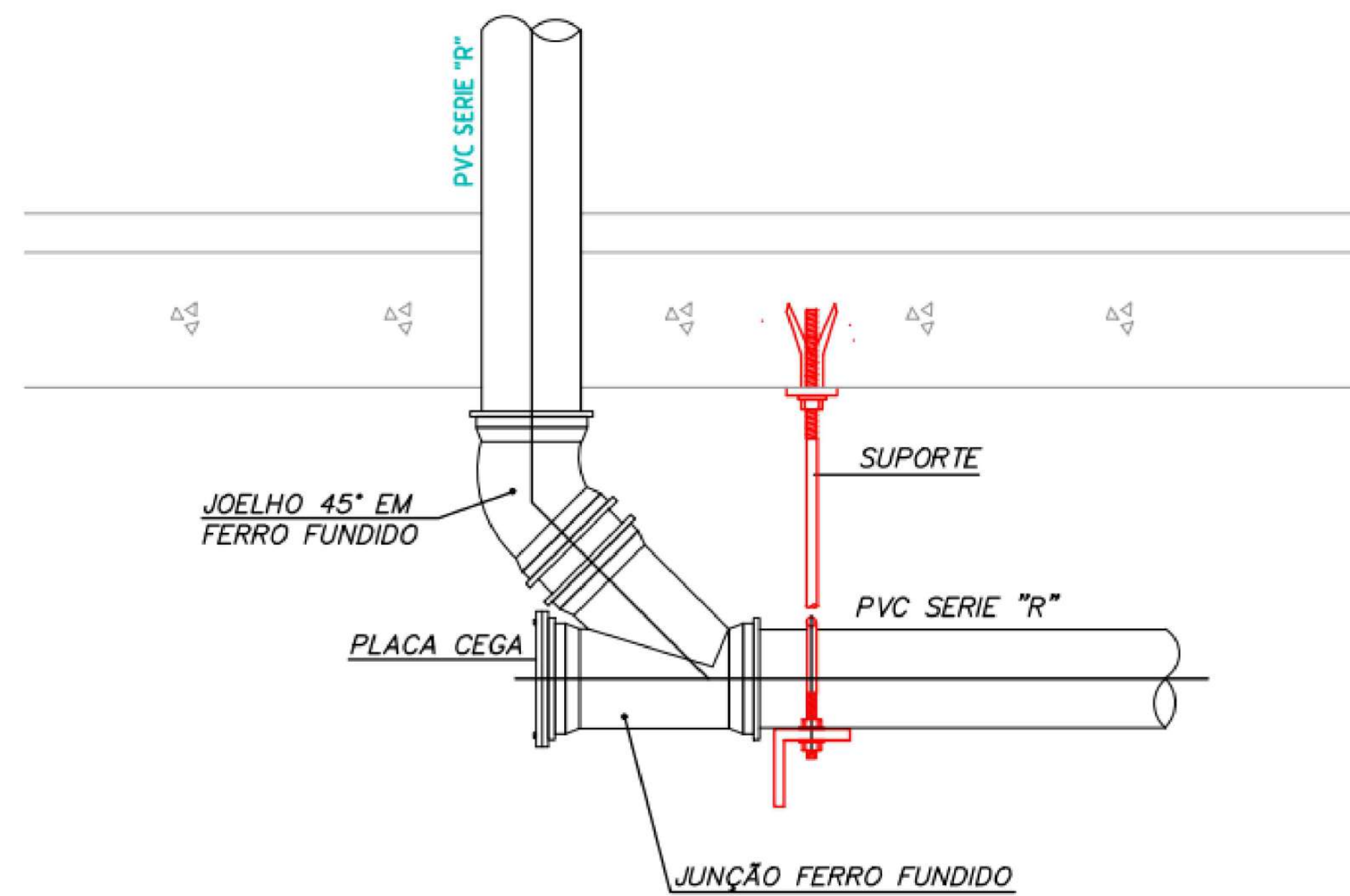
DETALHE DO PÉ DE COLUNA COM JUNÇÃO P/INSPEÇÃO SEM ESCALA
