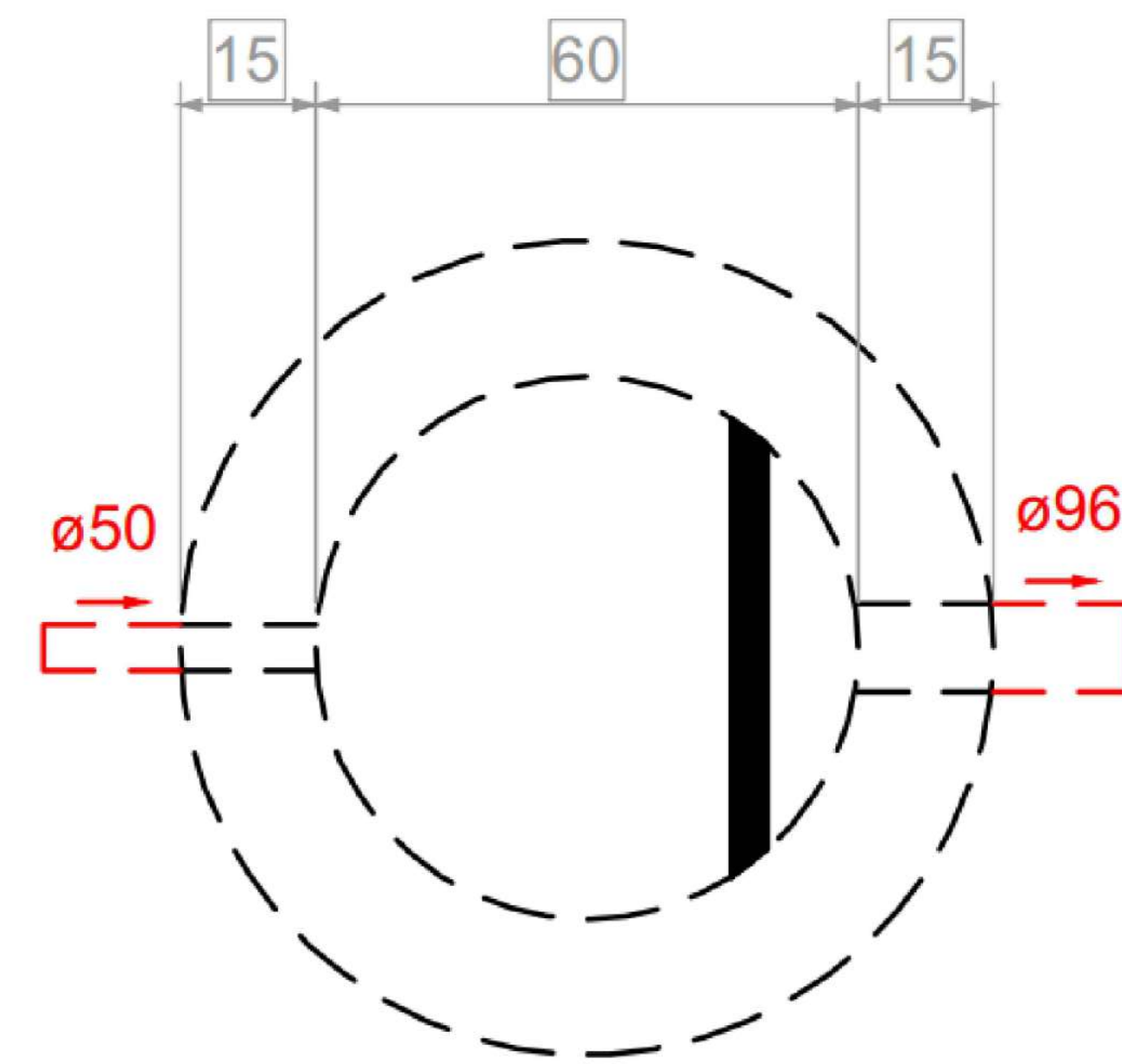
Caixa de gordura - TÉRREO Planta baixa - ESC. 1:25
