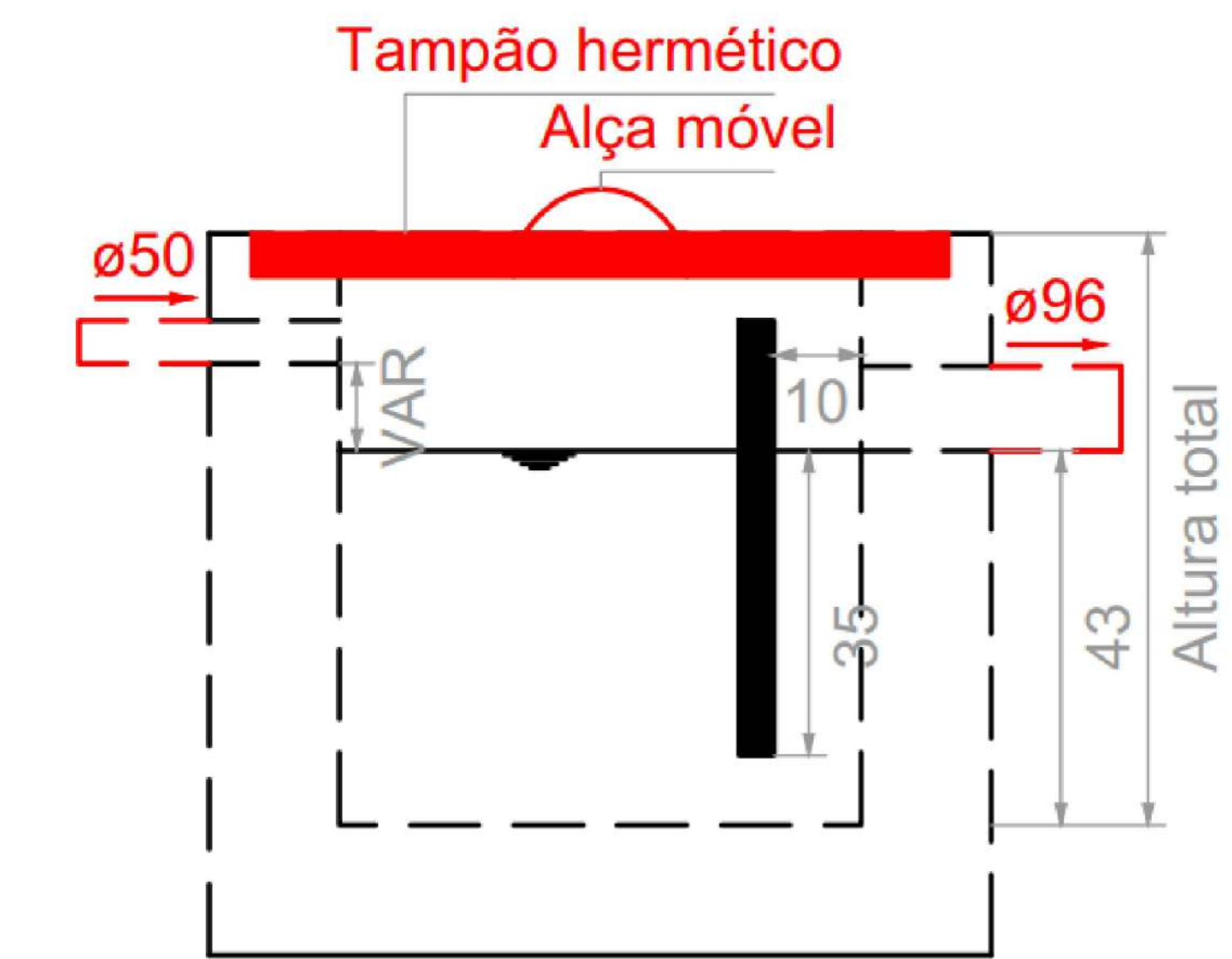
Caixa de gordura - TÉRREO Corte 1 - ESC. 1:25
