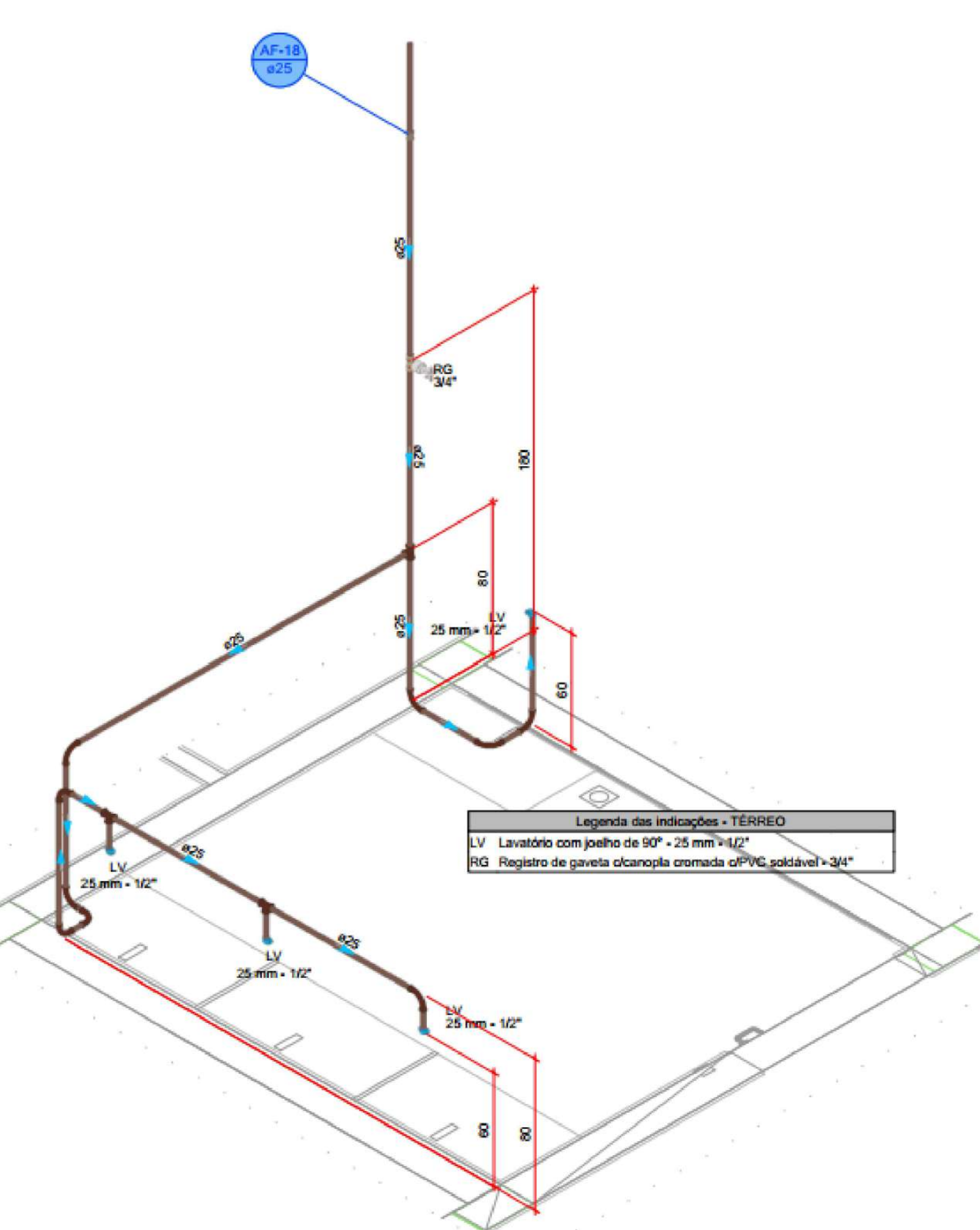
DETALHE HID-17 1:25
