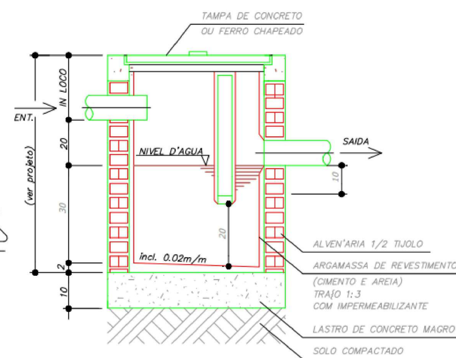
CORTE A-A
