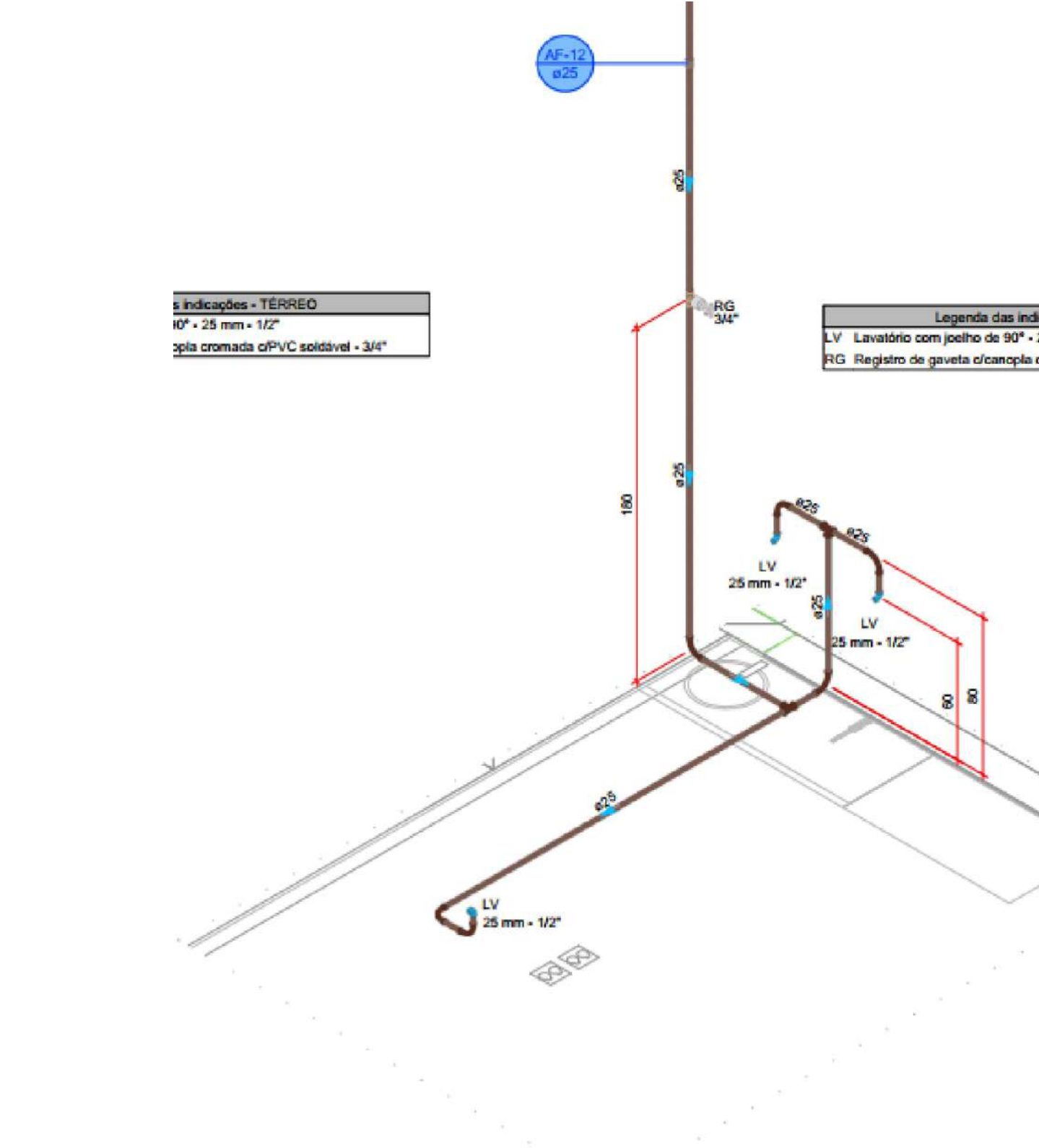
DETALHE HID-11=12=15=18=23 1:25
