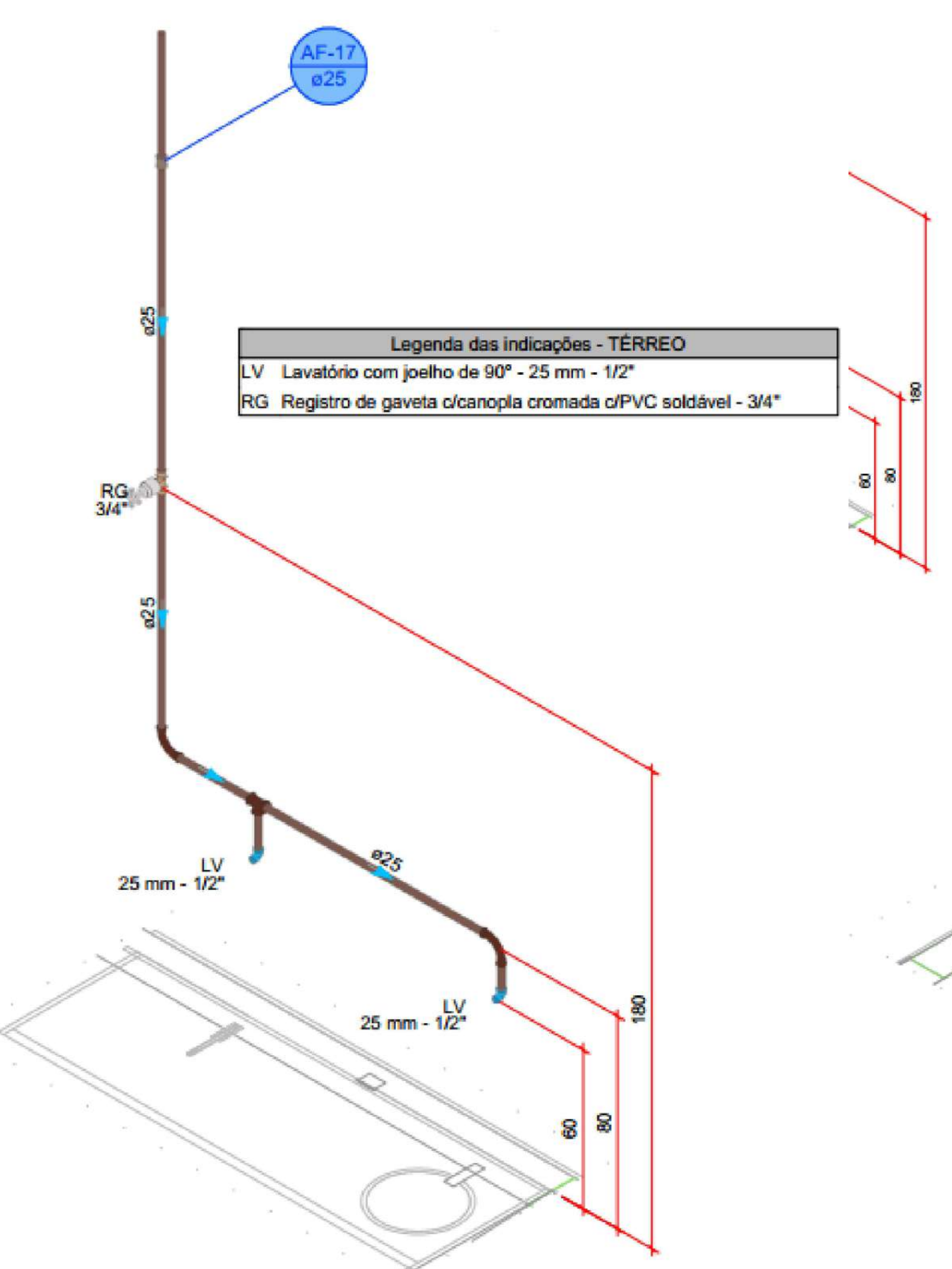
DETALHE HID-16 1:25
