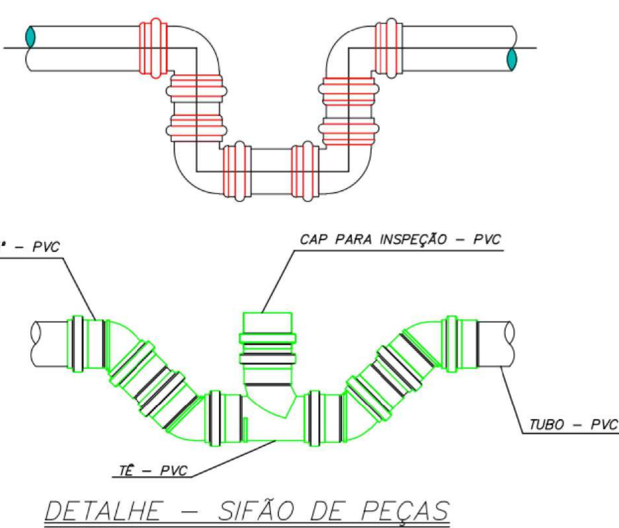
DETALHE - SIFÃO DE PEÇAS SEM ESCALA
