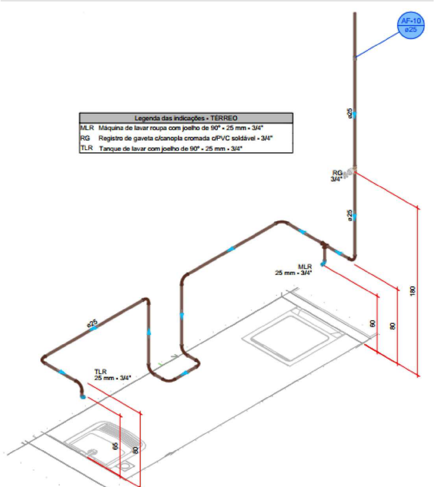
DETALHE HID-9 1:25
