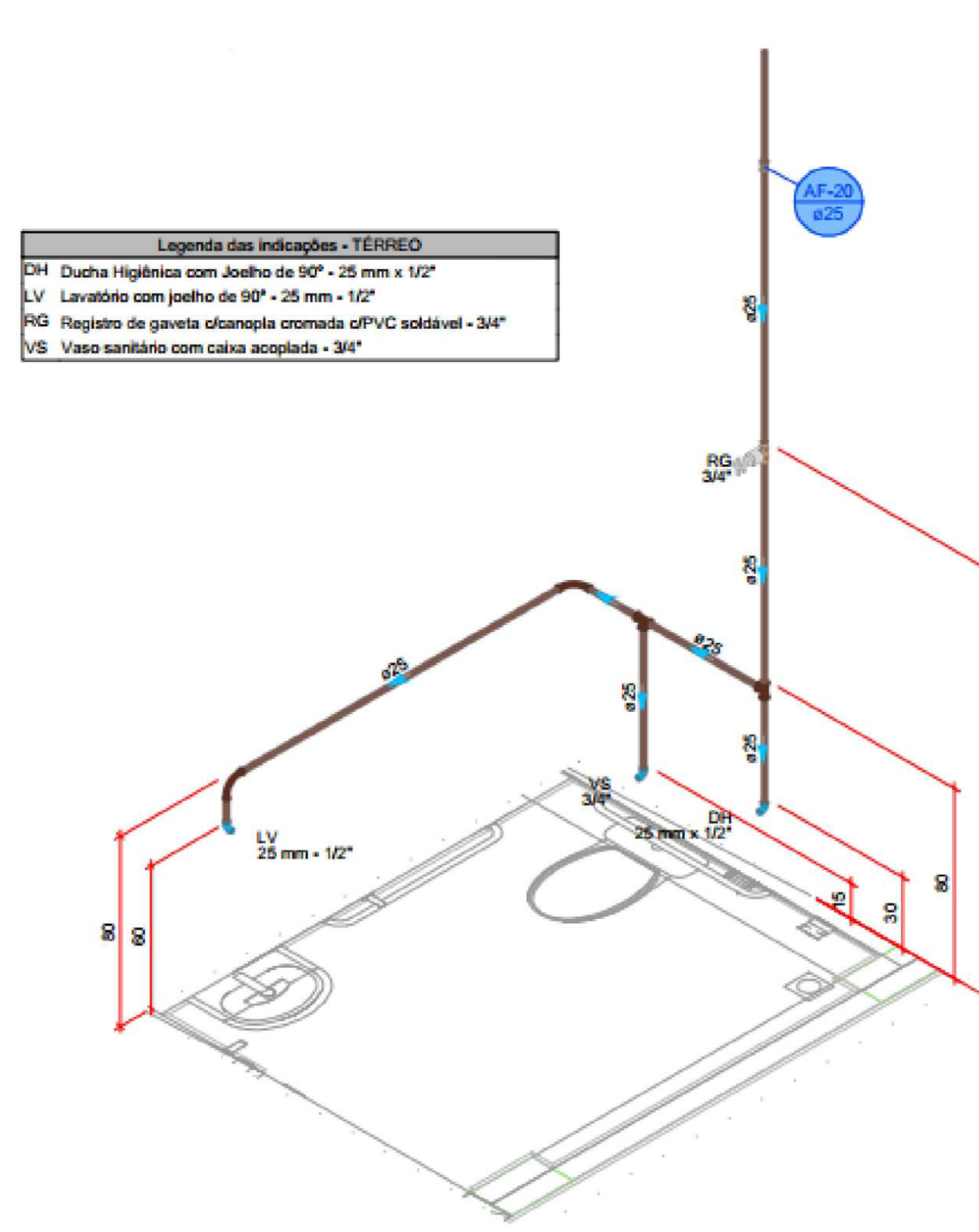
DETALHE HID-20 1:25
