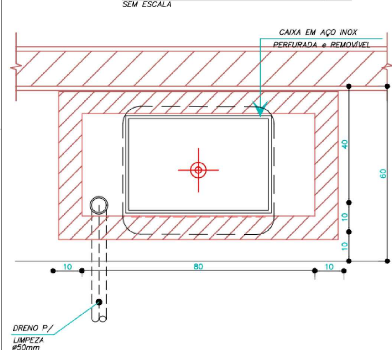
PLANTA BAIXA
