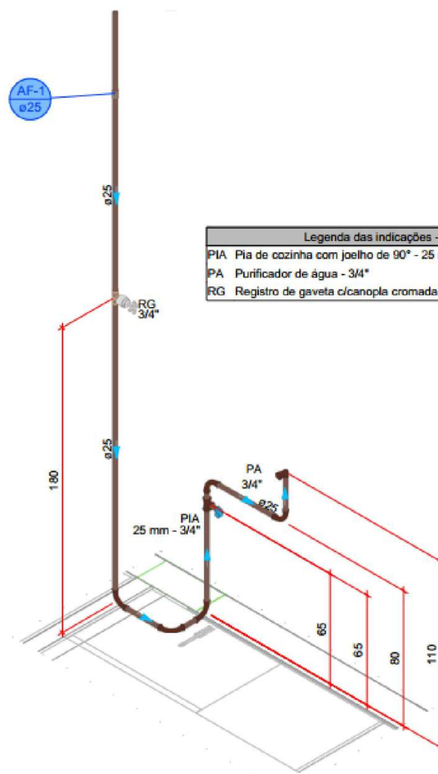
DETALHE HID-1 1:25
