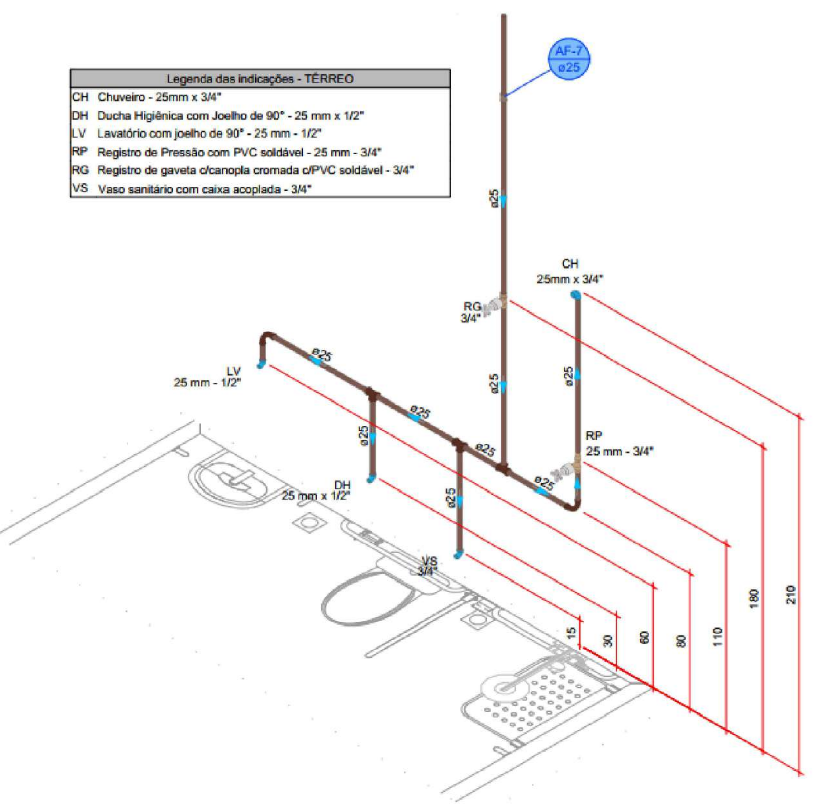
DETALHE HID-8 1:25
